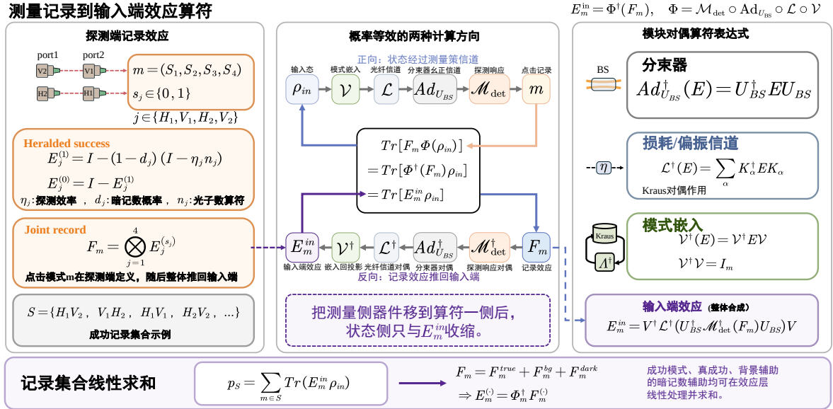
图 3.1 中间站测量侧的效应算符推回关系。探测端先构造点击记录 F_m , 再按探测器响应、分束器、光纤信道和模式嵌入的对偶顺序推回输入端, 得到用于收缩的 E_m^{in} 。状态侧输出 \rho_{in} 与该效应算符共同进入概率收缩。该处理与开放系统中的对偶信道表述一致 [51,63,64] 。
