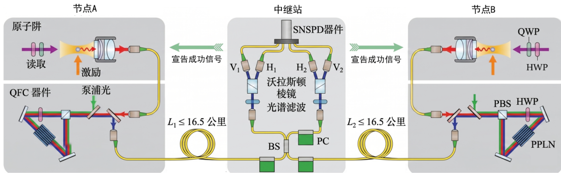
图 1.3 中性原子远程纠缠链路。节点 A 和节点 B 通过读出、激发与原子-光子接口产生链路光子，QFC 模块将原子波段光子转换到电信波段并经 L_1, L_2 \leq 16.5 \text{ km} 光纤送入中继站。中继站利用沃拉斯顿棱镜、光谱滤波、分束器、偏振分析和 SNSPD 完成部分 BSM，并向两端返回成功宣告。图中“宣告成功信号”表示 heralding signal。BS 为分束器，PBS 为偏振分束器，HWP/QWP 为半波片/四分之一波片，PPLN 为周期极化铌酸锂波导，SNSPD 为超导纳米线单光子探测器 [28,29,32-34] 。
