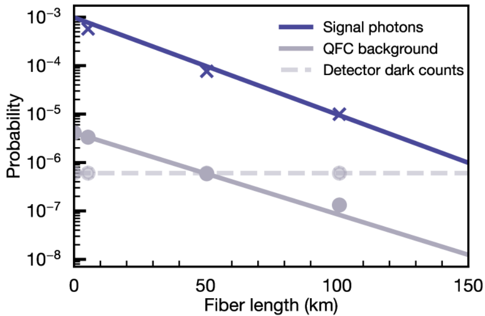
图 1.4 链路长度增加时信号与噪声相对变化的示意图。图片引自 Zhou 等关于处理节点量子网络链路噪声分析的工作 [33] 。
