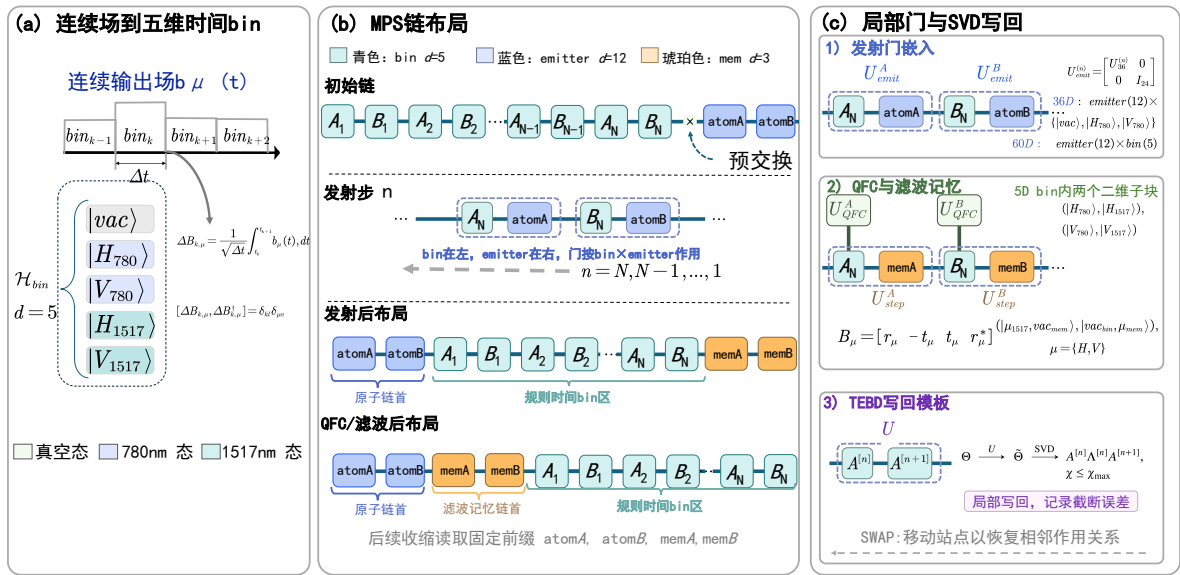
图 2.1 连续时间链路到 MPS/TEBD 计算对象的映射。连续输出场在时间步长 \Delta t 下离散为时间分箱。两臂发射体、时间分箱和滤波记忆模随后排列成一维 MPS 链。每个时间步由发射门、QFC 门、滤波记忆门、SWAP 调度和 SVD 回写组成。该结构把连续时间光场、有限带宽记忆和局域门更新统一到可收缩的张量网络表示中 [46,48,49,53-55] 。
