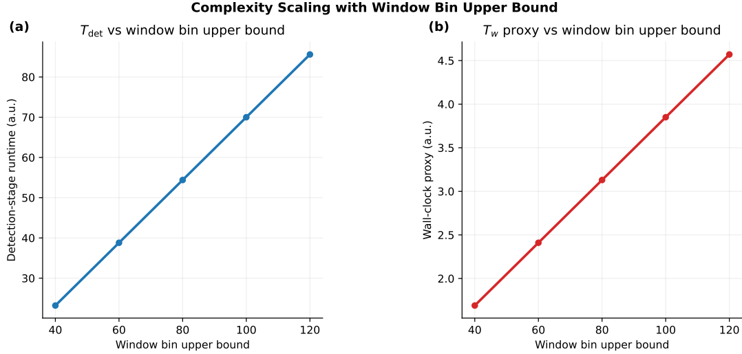
图 4-14 复杂度缩放图：(a) 探测阶段耗时随窗口 bin 数增长；(b) 墙钟代理量随 bin 个数上限增长。
