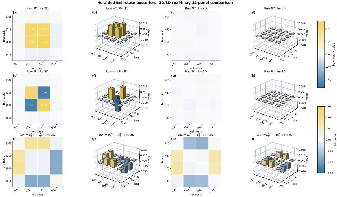
图 4-7 宣告成功条件下 Bell 后验态密度矩阵的十二联图：三行分别对应 raw \Psi^+ 、raw \Psi^- 与 \Delta\rho_H = \rho_H^+ - \rho_H^- ；每行四列依次为二维实部热图、三维实部柱图、二维虚部热图与三维虚部柱图。
