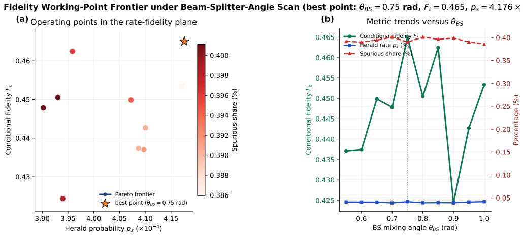
图 4-12 速率-保真度工作点前沿（分束器混合角扫描）：（a）每次尝试宣告概率与条件保真度的工作点平面，并以颜色表示假成功占比；（b）条件保真度、每次尝试宣告概率与假成功占比随 \theta_{BS} 的变化。
