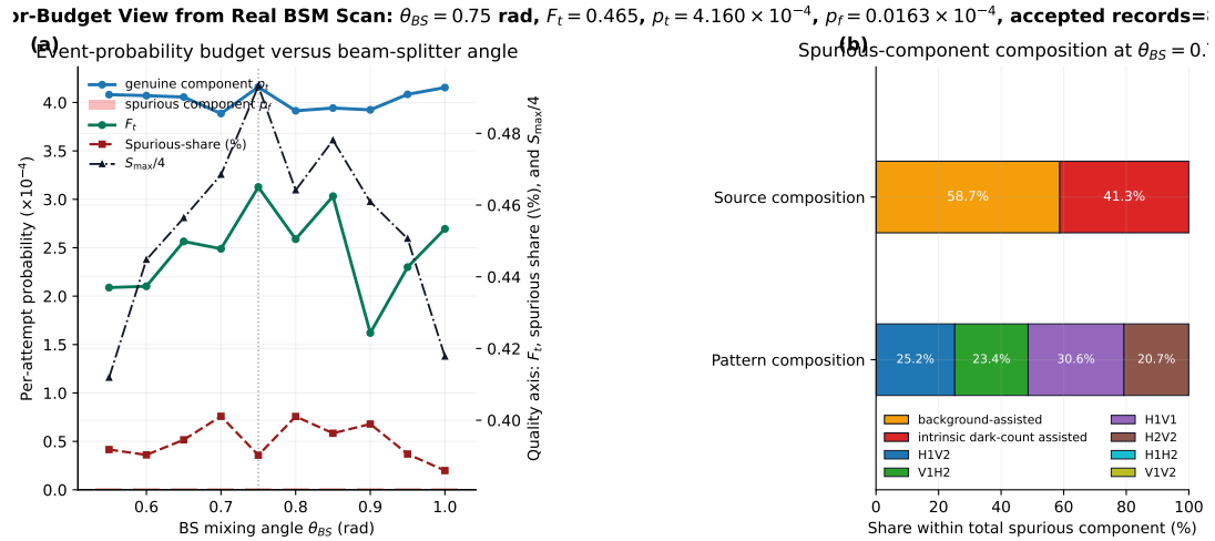
图 4-13 误差预算汇总图（真实 BSM 扫描）：（a）真成功/假成功宣告概率预算及 F_t 、假成功占比、 S_{\max}/4 随 \theta_{BS} 的联合变化；（b）推荐工作点的假成功来源（背景辅助与内禀暗计数辅助）及其模式贡献分解。
