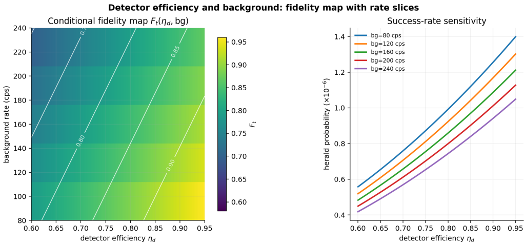
图 4-13 探测效率-背景联合扫描下的保真度热图与成功率切片。
