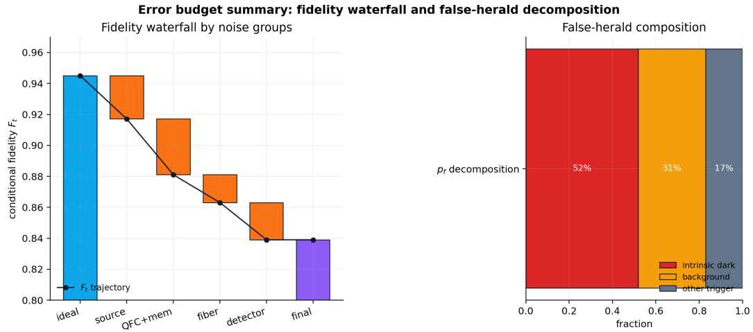
图 4-15 误差预算汇总图：左为按噪声组分解的条件保真度瀑布图，右为假成功事件组成分解。
