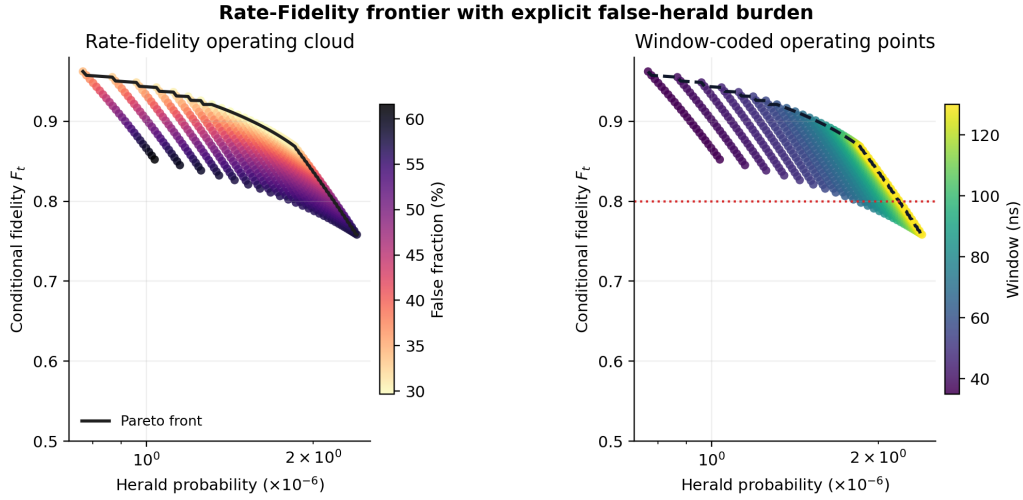
图 4-14 速率-保真度工作点前沿。
