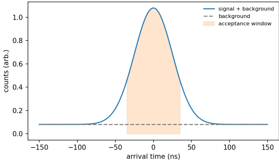
图 4-4 点击时间分布与接受窗口。
