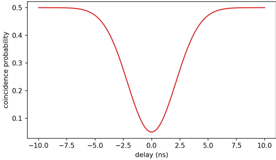
图 4-6 HOM 曲线及可见度约束。
