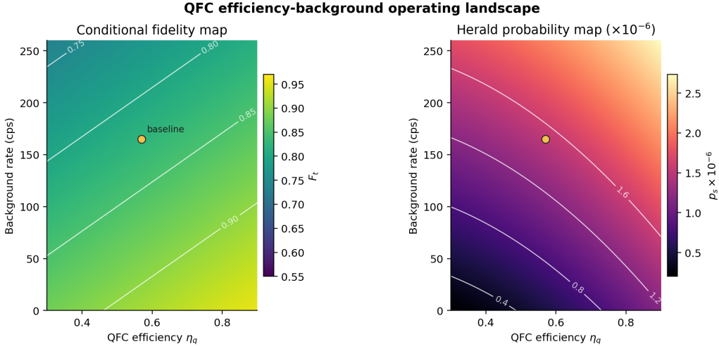
图 4-12 QFC 背景噪声对事件率与保真度的影响。
