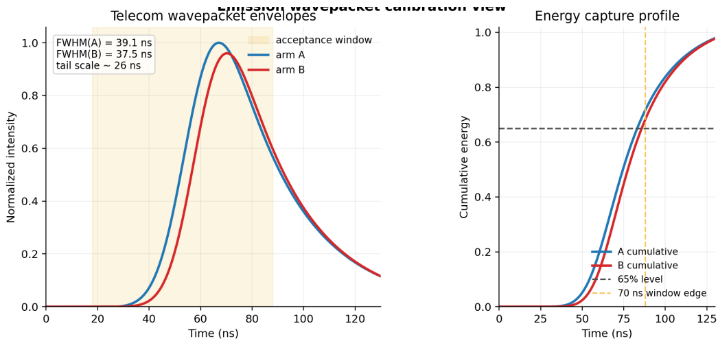
图 4-2 双臂波包时域结构与主窗口位置。
