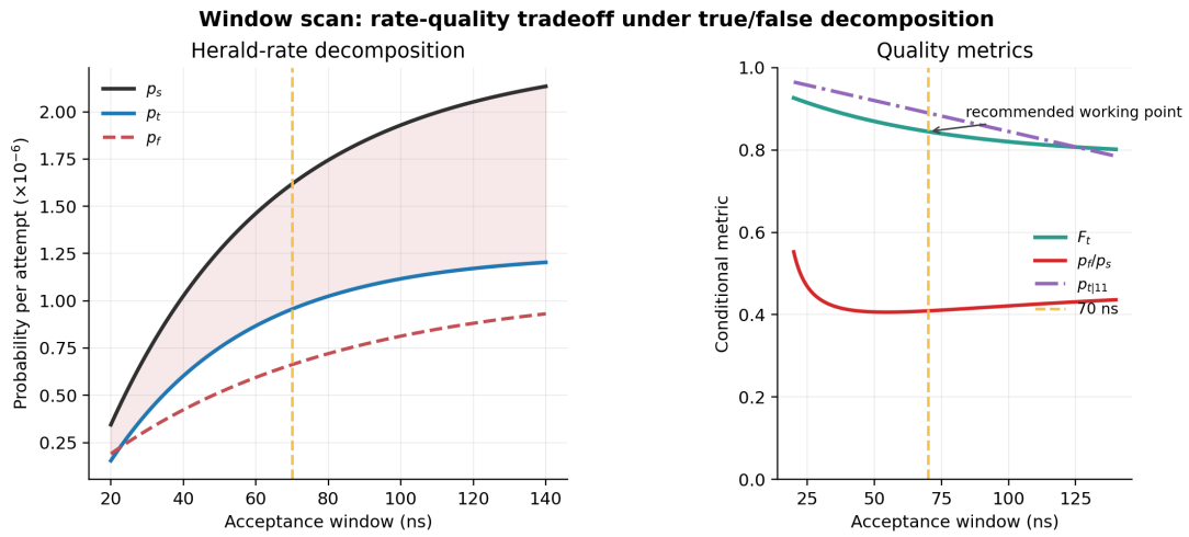
图 4-5 窗口扫描下的速率、条件保真度与假成功占比。
