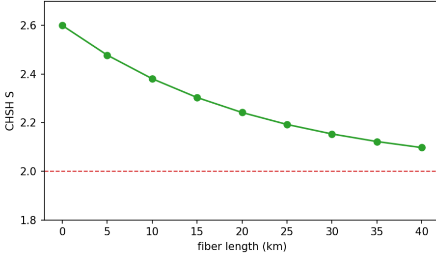
图 4-10 CHSH 参数趋势（虚线为经典界 S = 2 ）。
