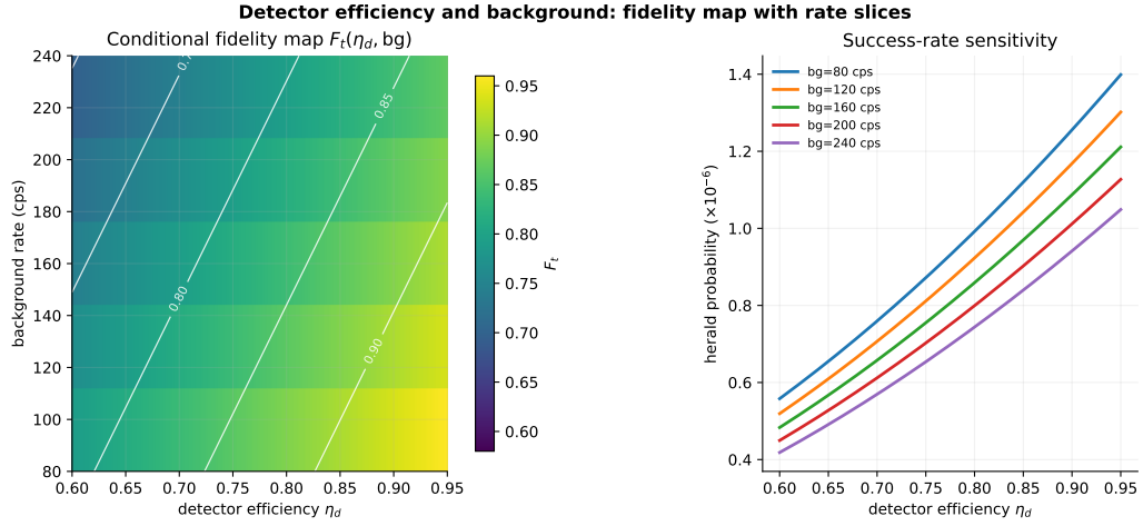
图 4-12 探测效率-背景联合扫描下的保真度热图与成功率切片。
