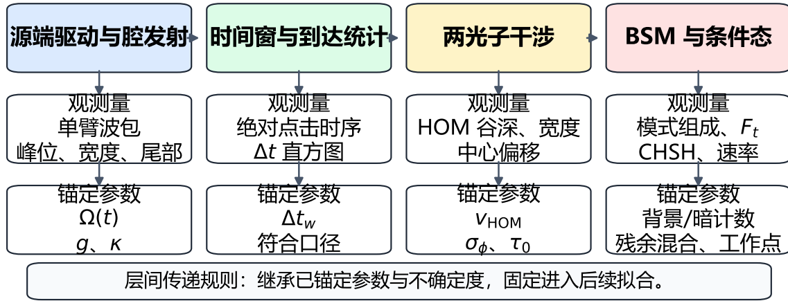
图 4.1 按装置环节组织的分层标定图：从源端发射、时间窗、HOM 干涉到 BSM 与条件态，每一层只用本层观测量锚定对应参数，并把约束传递到下一层。
