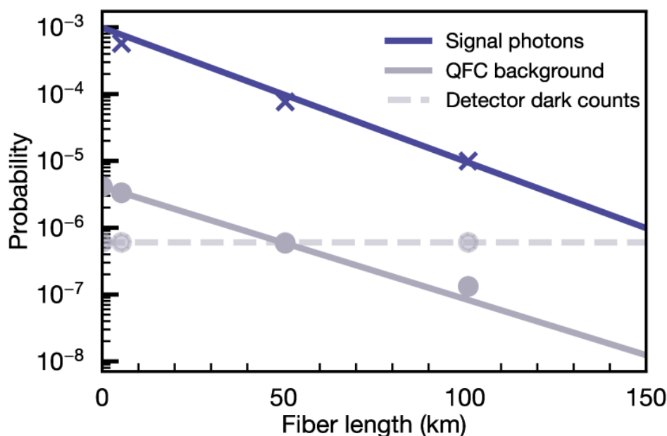
图 1.6 链路长度增加时信号与噪声的相对变化示意图。随着距离增加，真实信号计数率指数衰减，而暗计数和部分背景噪声近似保持在固定本底，系统因此会从效率受限逐渐转向噪声受限。该现象提示接口评估不能只做链路损耗预算，而需要把背景与暗计数纳入同一统计框架。图片引自 Zhou 等关于处理节点量子网络链路噪声分析的工作。 [31]
