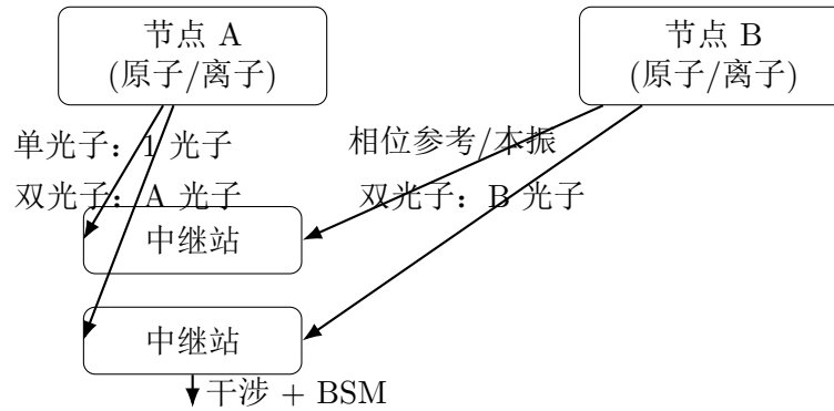
图 1.3 单光子与双光子干涉型远程纠缠方案示意图。单光子方案对相位参考更敏感但成功率可线性受益于链路效率；双光子方案把相位稳定需求更多局域到中继站，更适合长光纤部署，但成功率对两边链路效率更敏感。图示据相关文献思路整理绘制。 [24-25,27]
