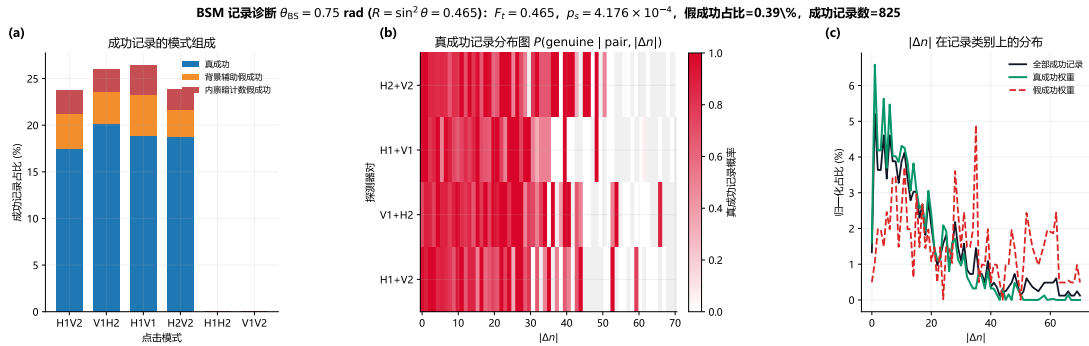
图 4.6 基于真实 BSM 扫描汇总结果的三联诊断图：(a) 推荐工作点 ( \theta_{BS} = 0.75 \text{ rad} ) 下宣告记录在各点击模式上的后验组成（真成功、背景辅助假成功、内禀暗计数辅助成功）；(b) 探测器对与相对时间仓索引差 |\Delta n| 的记录真实性热图；(c) 总成功、真成功与假成功三类权重在 |\Delta n| 上的归一化分布。
