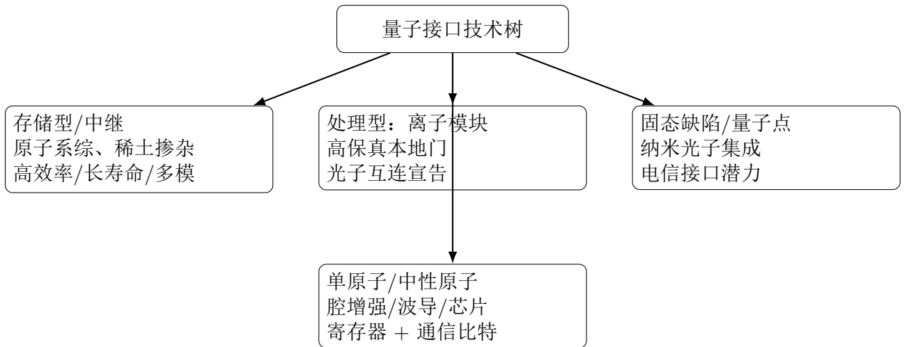
图 1.4 典型量子接口平台的技术树与优缺点概览。图示据相关文献思路整理绘制。 [12-13,28-29,35-37]
