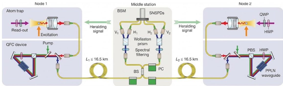
图 1.5 所研究的端到端链路示意图：两端 ^{87}\text{Rb} 原子在腔增强条件下产生原子-光子纠缠；光子经量子频率转换（QFC）转到电信波段并通过长光纤发送至中间站；中间站通过两光子干涉与部分贝尔态测量（BSM）宣告远程原子贝尔对。 [21-22,43,47-48]
