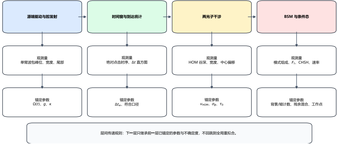
图 4.1 按装置环节组织的分层标定图：从源端发射、时间窗、HOM 干涉到 BSM 与条件态，每一层只用本层观测测量锚定对应参数，并把约束传递到下一层。
