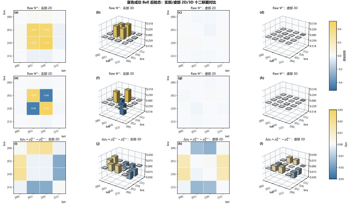
图 4.6 宣告成功条件下 Bell 后验态密度矩阵的十二联图：三行分别对应 \text{raw } \Psi^+ 、 \text{raw } \Psi^- 与 \Delta\rho_{\text{ff}} = \rho_{\text{ff}}^+ - \rho_{\text{ff}}^- ；每行四列依次为二维实部热图、三维实部柱图、二维虚部热图与三维虚部柱图。
