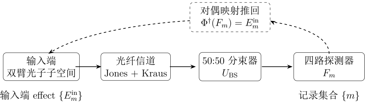
图 3.2 中间站测量侧的 effect 推回关系。探测端先构造点击记录 F_m ，再经光纤信道和分束器的对偶映射推回输入端，得到用于收缩的 E_m^{\text{in}} 。这一路径保留了损耗、偏振旋转和探测器响应，又避免在态端重复施加线性光学网络。该处理与开放系统中的对偶信道表述一致 [40,52-53] 。
