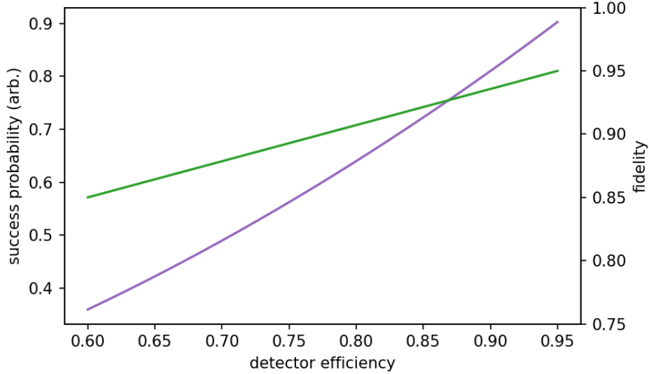
图 4-6 探测器效率对成功率与保真度的影响
