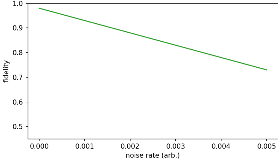
图 4-4 保真度随噪声率变化
