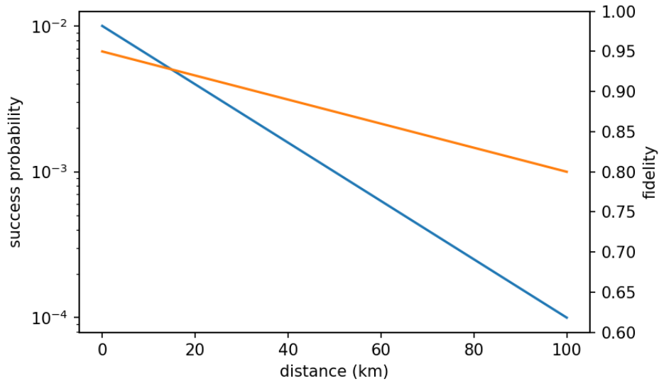
图 4-5 成功率与保真度随光纤长度变化
