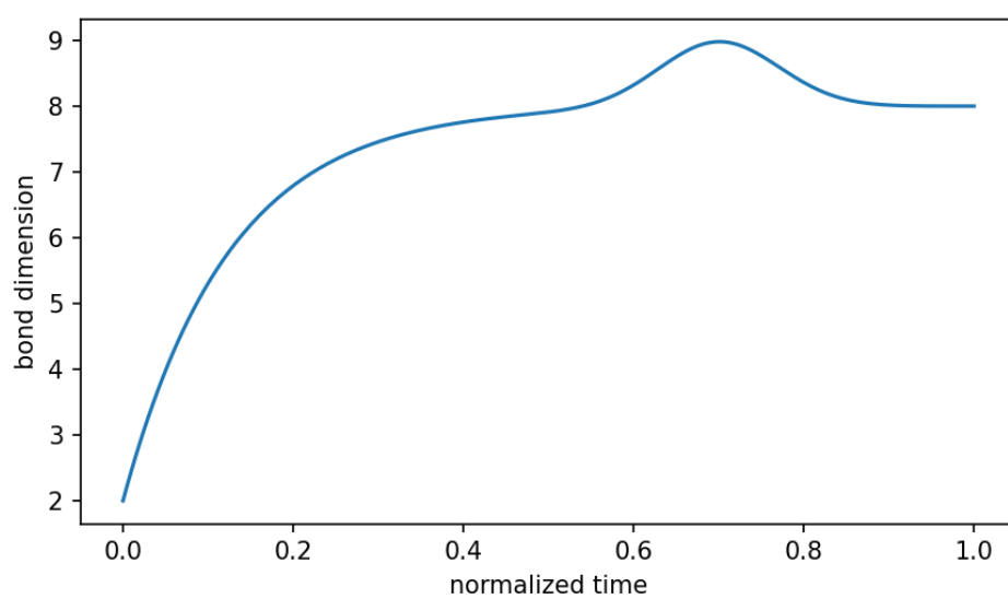
图 4-2 发射过程中 MPS 键维度的演化
