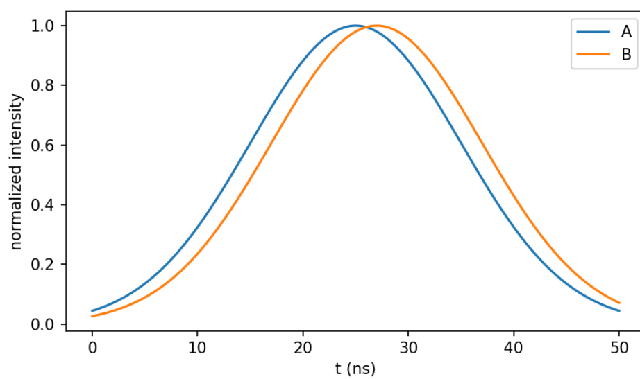
图 4-1 发射波包时间结构
