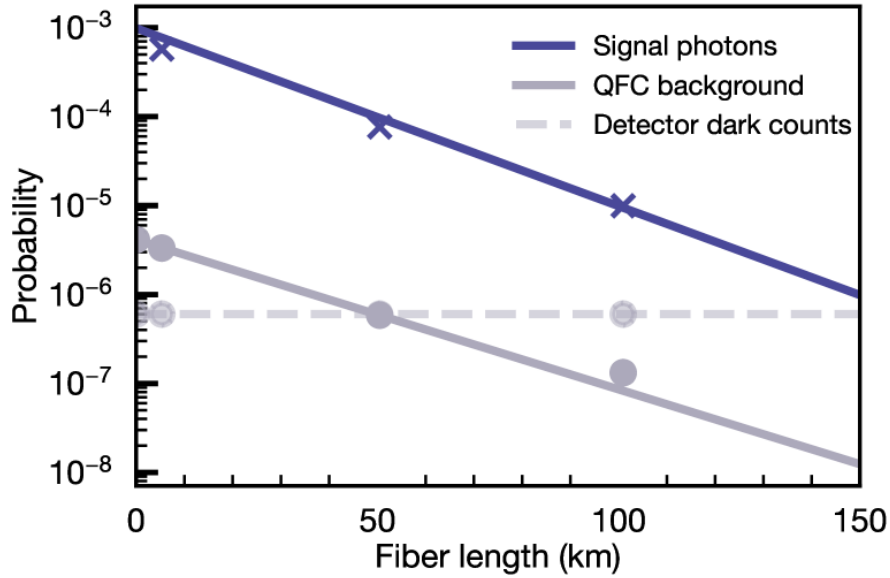
图 1-6 链路长度增加时信号与噪声的相对变化示意图。随着距离增加，真实信号计数率指数衰减，而暗计数和部分背景噪声近似保持在固定本底，系统因此会从效率受限逐渐转向噪声受限。该现象提示接口评估不能只做链路损耗预算，而需要把背景与暗计数纳入同一统计框架。图片引自 Zhou 等关于 processing-node 量子网络链路噪声分析的工作。 [29]
