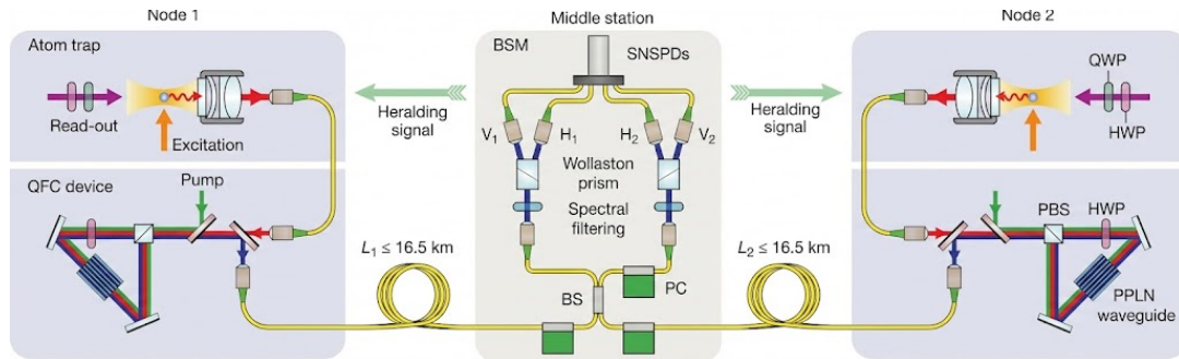
图 1-5 本文关注的端到端链路示意图: 两端 ^{87}\text{Rb} 原子在腔增强条件下产生原子-光子纠缠; 光子经量子频率转换 (QFC) 转到电信波段并通过长光纤发送至中间站; 中间站通过两光子干涉与部分 Bell 态测量 (BSM) 宣告远程原子 Bell 对。 [19,20,41,45,46]
