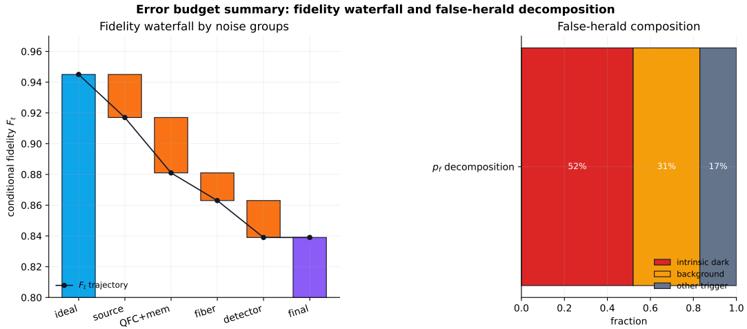
图 4-14 误差预算汇总图：左为按噪声组分解的条件保真度瀑布图，右为假成功事件组成分解。
