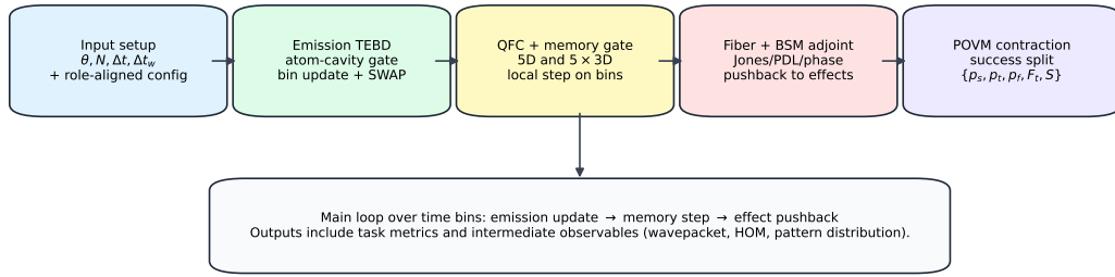
图 3-1 端到端单次任务仿真流程图：从参数与离散设置输入，经发射 TEBD、QFC+ 记忆门、光纤与 BSM 对偶推回、POVM 收缩，输出任务指标与中间可观测量。
