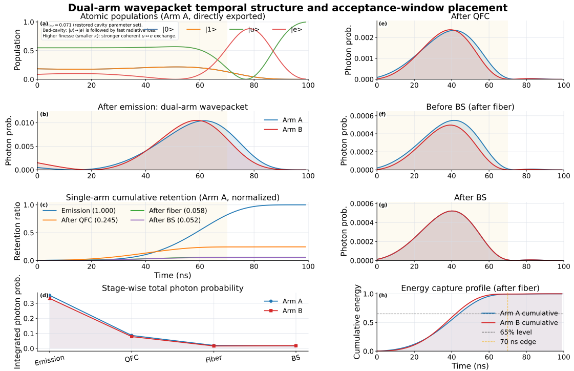
图 4-2 双臂波包时域结构与主窗口位置：(a) A 臂原子四能级占据演化；(b) 发射后双臂波包；(c) A 臂累计保留率；(d) 各阶段总光子概率积分；(e) QFC 后双臂波包；(f) 光纤后、入 BS 前波包；(g) BS 后波包；(h) 光纤后累计能量捕获。
