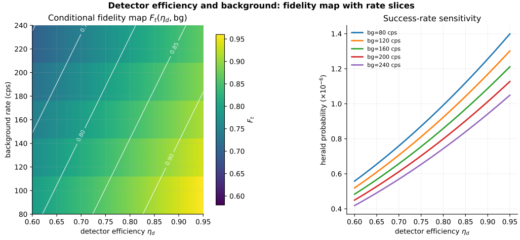
图 4-12 探测效率-背景联合扫描下的保真度热图与成功率切片。
