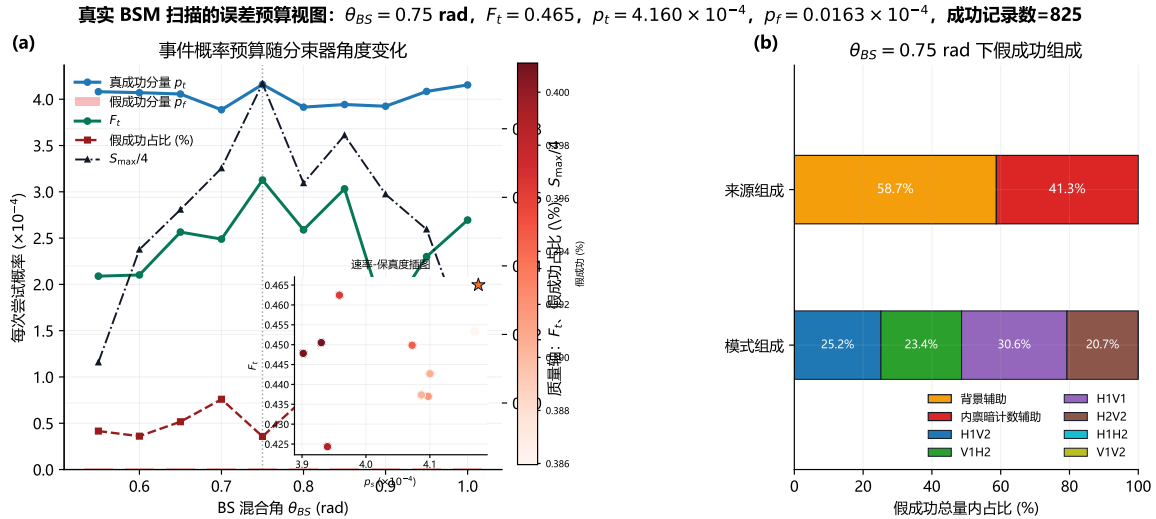
图 4.12 误差预算汇总图：(a) 真成功/假成功宣告概率预算及 F_t 、假成功占比、 S_{\text{max}}/4 随 \theta_{BS} 的联合变化（右下角 inset 为速率-保真度工作点前沿，颜色表示假成功占比）；(b) 推荐工作点的假成功来源（背景辅助与内禀暗计数辅助）及其模式贡献分解。
