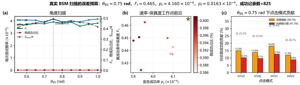
图 4.12 误差预算汇总图：(a) 真成功/假成功宣告概率预算及 F_t 、假成功占比、 S_{\max}/4 随 \theta_{BS} 的联合变化；(b) 速率-保真度工作点前沿，颜色表示假成功占比，星标表示推荐工作点；(c) 推荐工作点下各有效点击模式对假成功总量的贡献分解，并按来源并列给出背景辅助与内禀暗计数分量。
