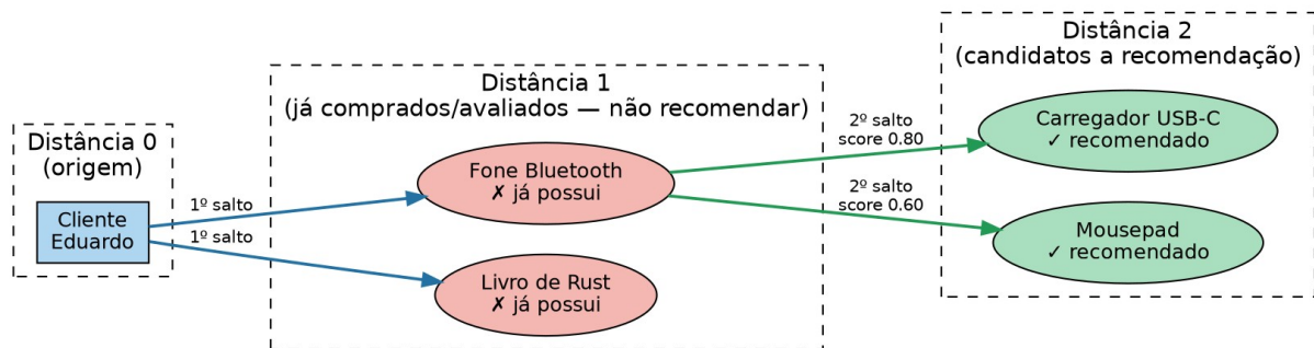
Figura 6 — Percurso BFS por camadas de distância a partir de um cliente. Fonte: elaborado pelo autor a partir do exemplo de recommend() em src/recommend.rs
