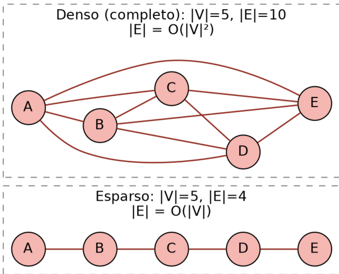
Figura 4 — Grafo esparsa × grafo denso (completo), para o mesmo número de vértices. Fonte: elaborado pelo autor
