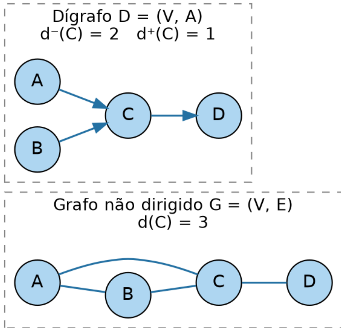
Figura 1 — Grafo não dirigido \times dígrafo, com grau, grau de entrada e grau de saída. Fonte: elaborado pelo autor
