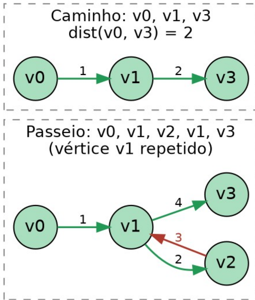
Figura 2 — Passeio (com vértice repetido) \times caminho, e distância entre dois vértices. Fonte: elaborado pelo autor
