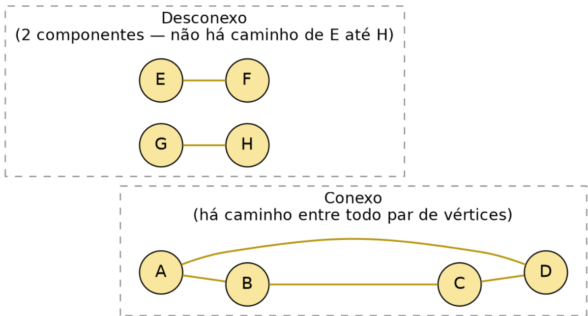
Figura 3 — Grafo conexo × grafo desconexo (com dois componentes). Fonte: elaborado pelo autor
