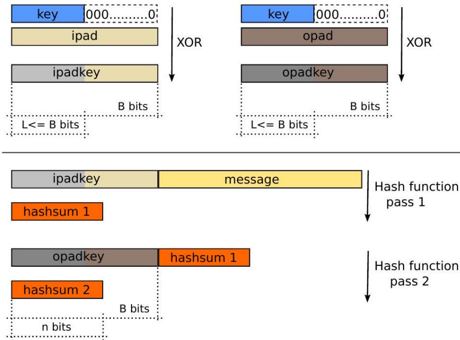
Fig. 5.5 Generating an HMAC (Source : Wikimedia Commons I)
