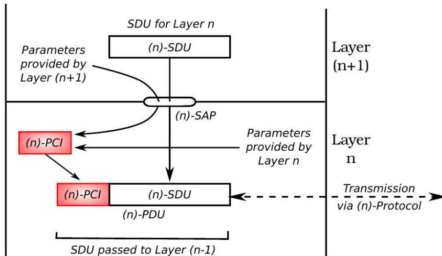
Fig. 6.3 Adding PCI to a PDU.
