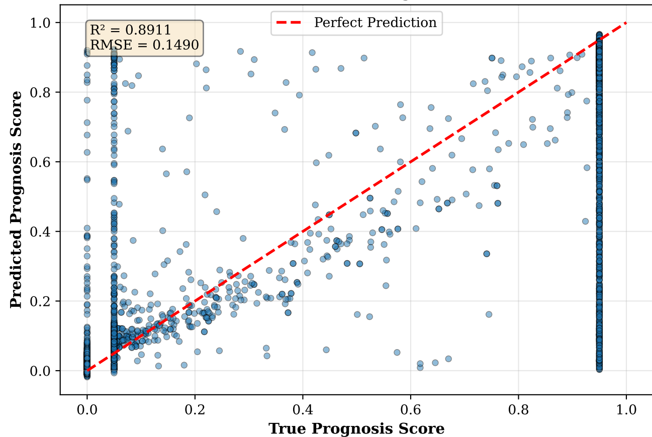
Predicted vs Actual Prognosis Scores
