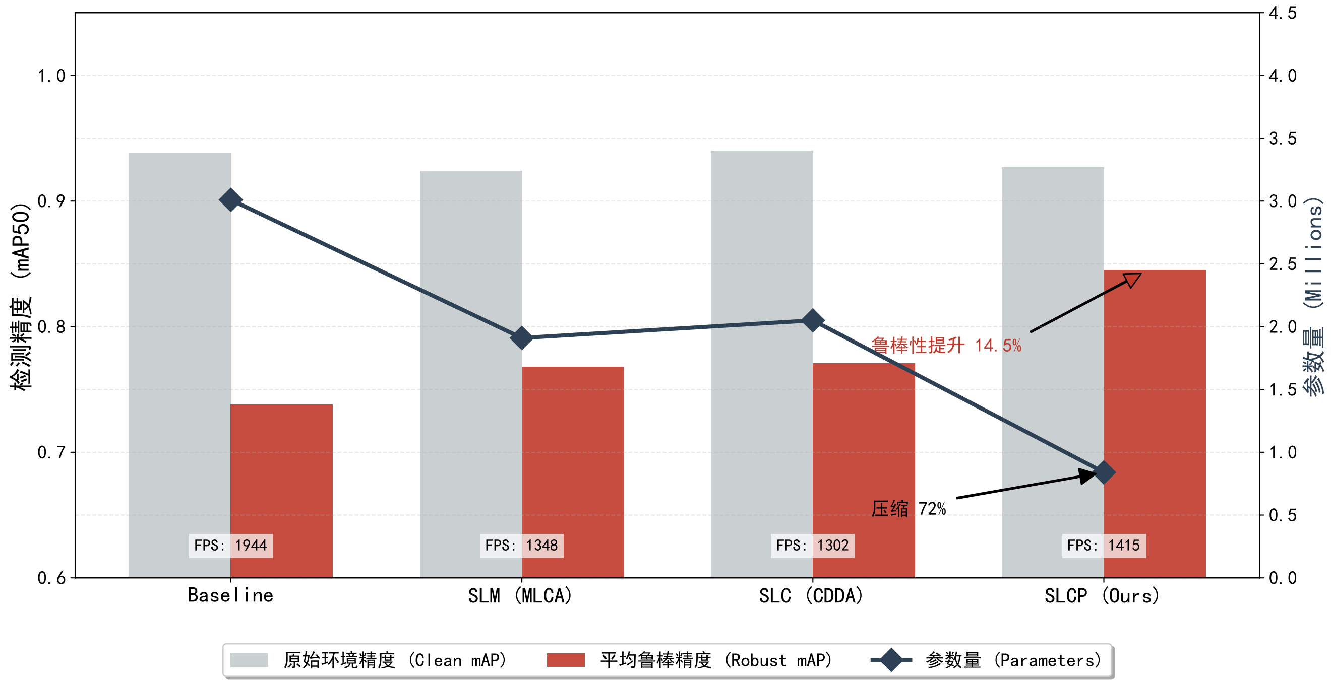
各阶段改进模型性能与效率综合对比分析
