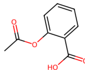
aspirin
