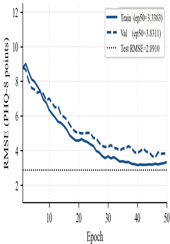
Audio Only (Wav2Vec2 + BiLSTM)
