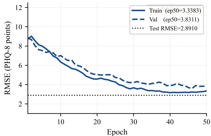
Audio Only (Wav2Vec2 + BiLSTM)
