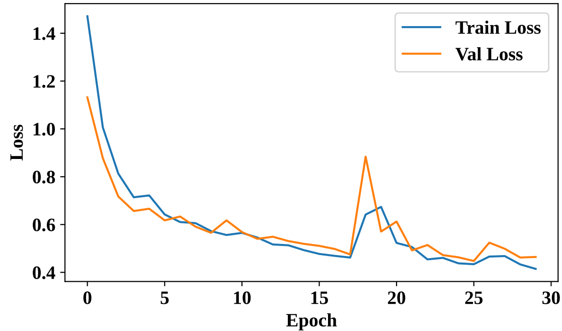
SimpleRNN: Loss
