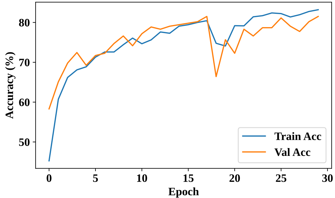
SimpleRNN: Accuracy
