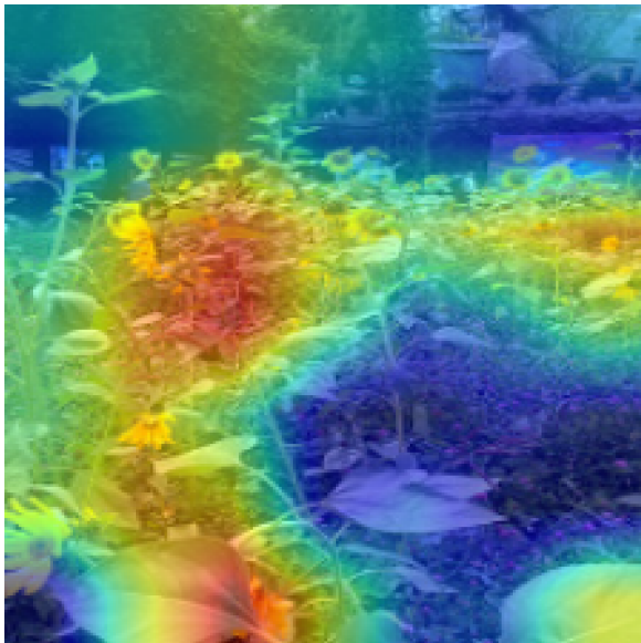
pred: tulips (1.00)
