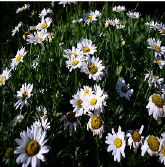
Input daisy
