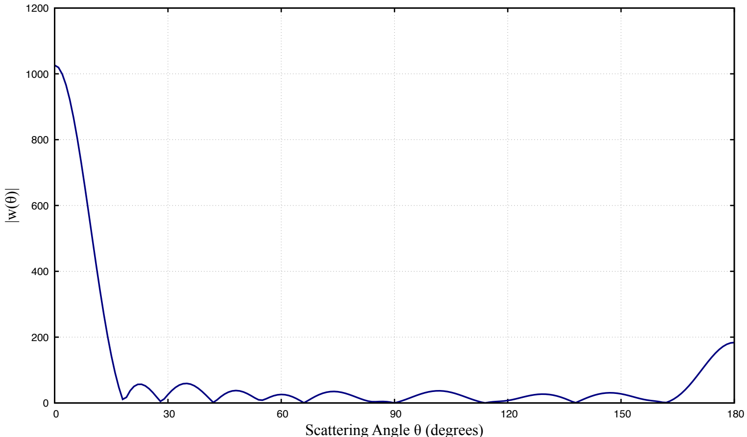
H+Xe: Magnitude |w(\theta)| ( l=7 )
