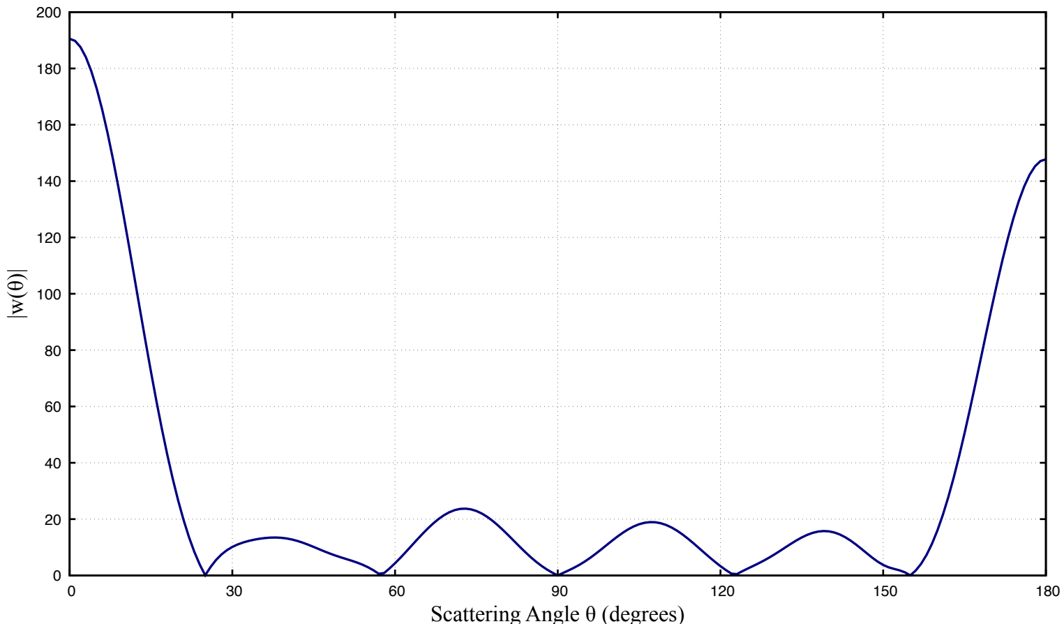
H+Xe: Magnitude |w(\theta)| ( l=5 )
