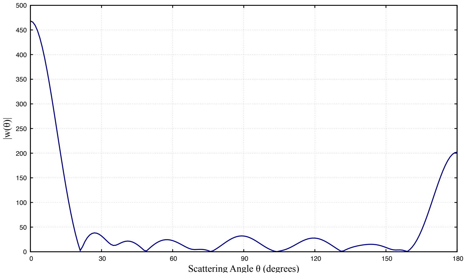
H+Xe: Magnitude |w(\theta)| ( l=6 )
