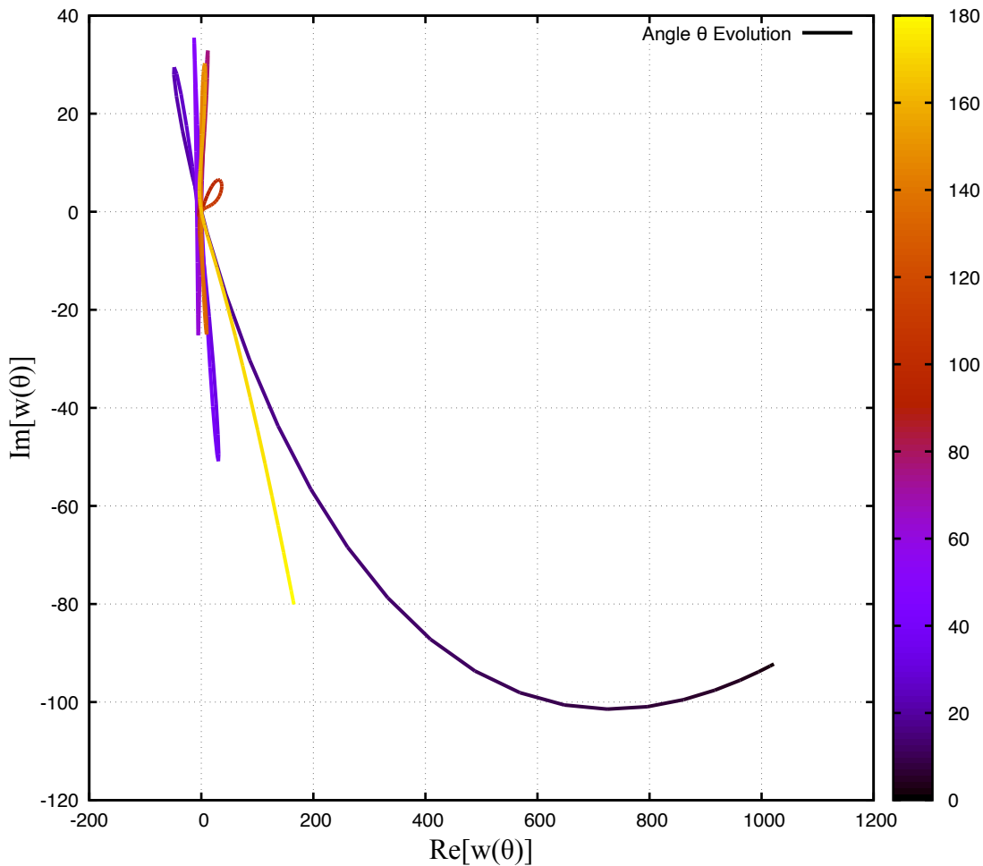
H+Xe: Complex w(\theta) Parameter Trajectory ( l=7 )
