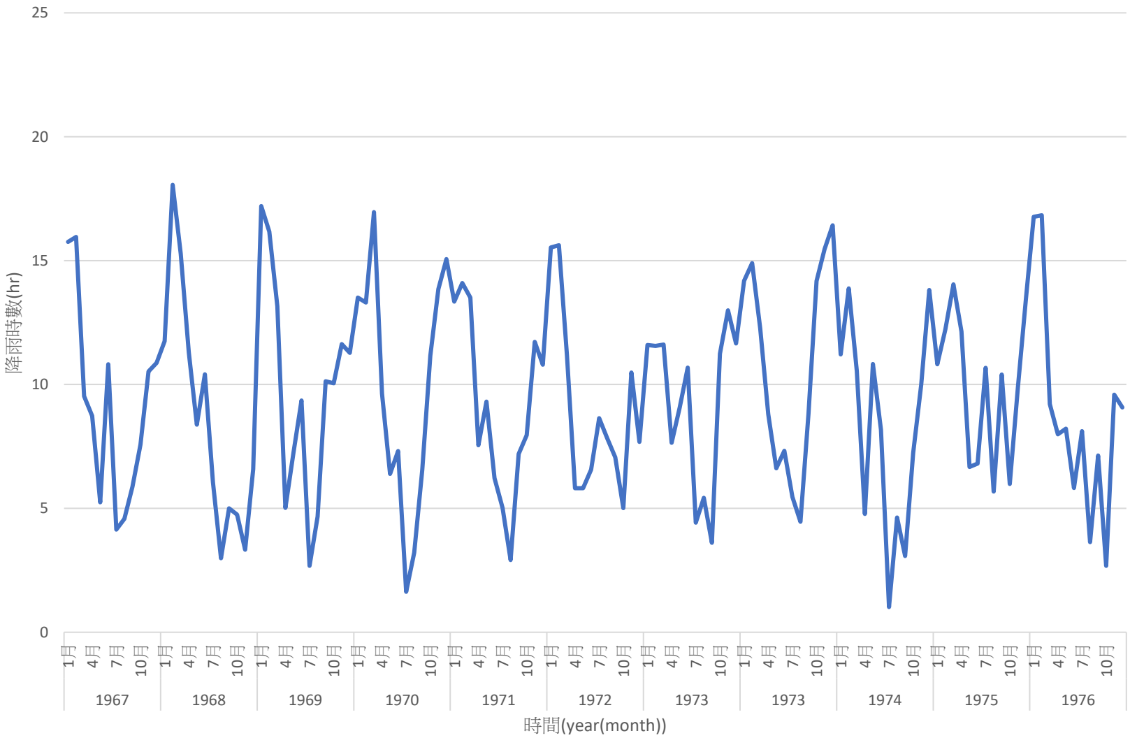
1967~1976降雨時數
