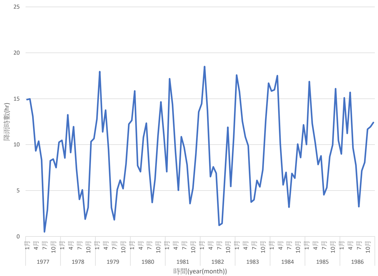
1977~1986降雨時數
