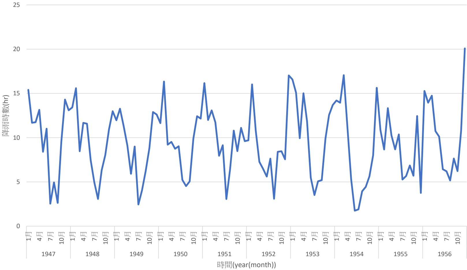
1947~1956降雨時數
