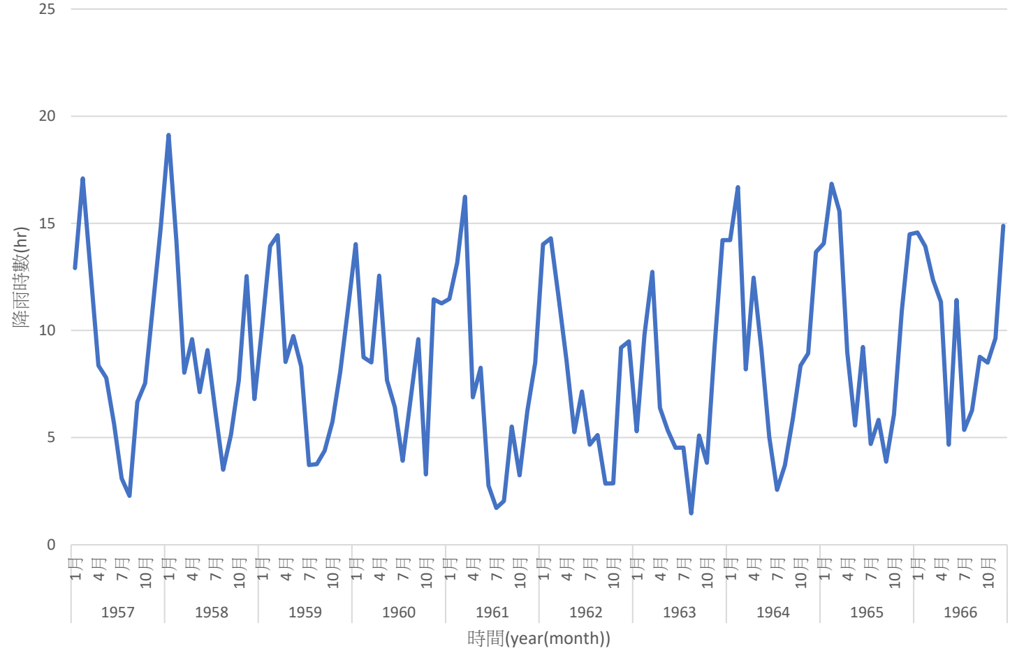
1957~1966降雨時數
