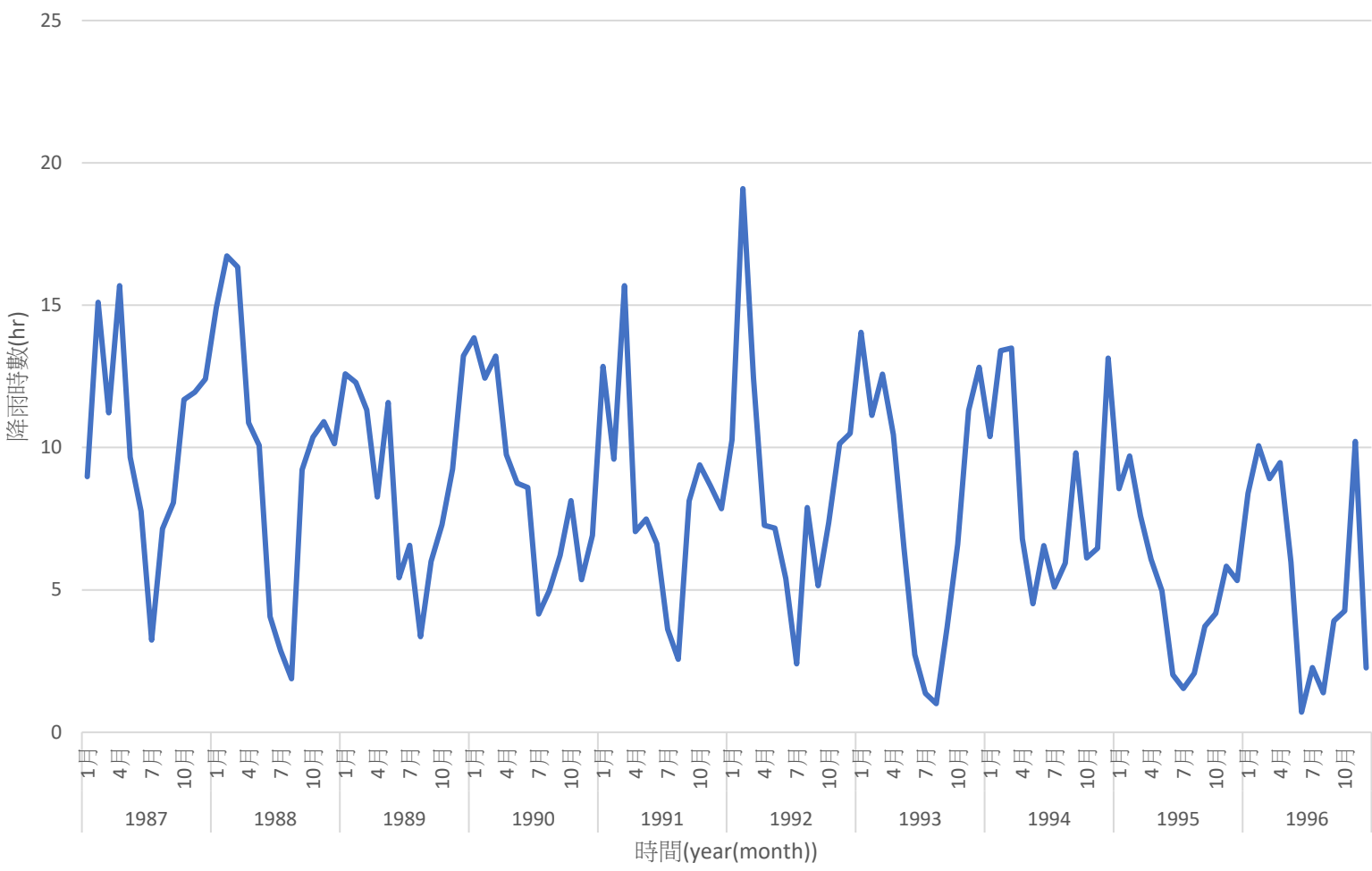
1987~1996降雨時數
