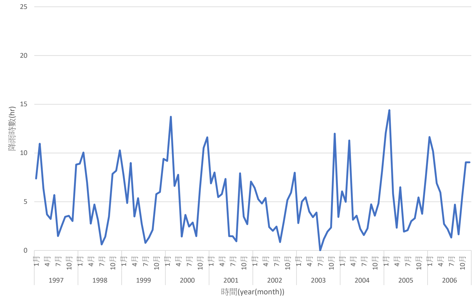
1997~2006降雨時數
