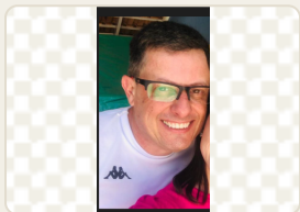
cassandro.png
