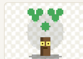
inimigo-ent.png
