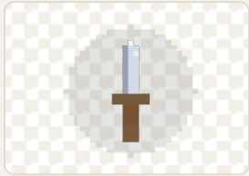
item-adaga.png
