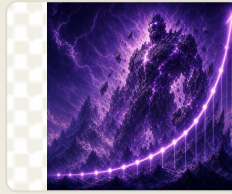
fase-complexidade.png
