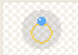
item-anel.png
