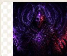
fase-lorde-segfault.png
