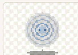
inimigo-eco.png
