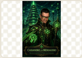
mestre-cassandro.png
