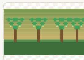
fundo-floresta.png
