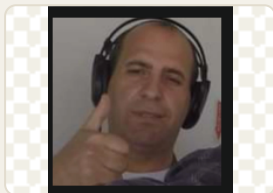
cesar.png
