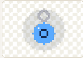
item-amuleto.png
