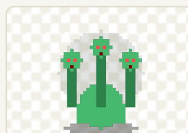
inimigo-hidra.png
