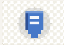
item-escudo.png
