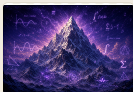
fundo-montanha.png
