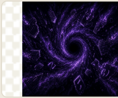
fase-abismo-devnull.png
