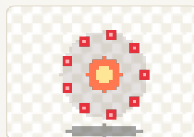
inimigo-ddos.png
