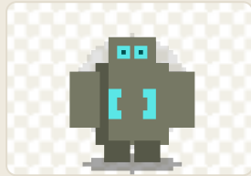
inimigo-golem.png
