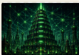
fundo-torre.png
