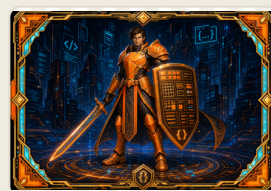
hud-guerreiro.png
