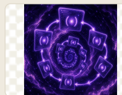
fase-recursao-limites.png
