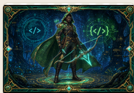
hud-ranger.png
