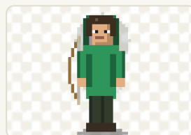
heroi-ranger.png
