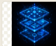
fase-padrao-mvc.png
