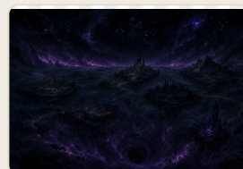
fundo-mapa.png
