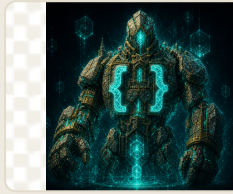
fase-classes-objetos.png
