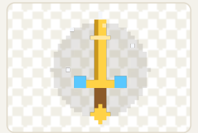
item-espada-lendaria.png
