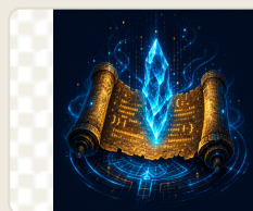
fase-prologo-despertar.png
