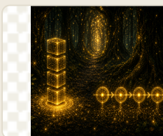
fase-pilhas-filas.png
