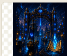
fase-porto-chegada.png
