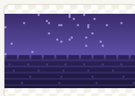
fundo-batalha.png
