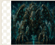
fase-god-class.png
