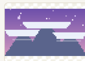
fundo-montanha.png
