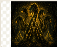
fase-hidra-recursiva.png
