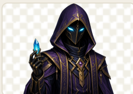
npc-narrador.png
