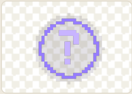
placeholder.png
