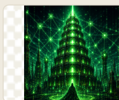
fase-torre-chegada.png
