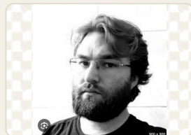
willen.png
