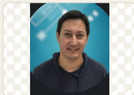
clayton.png
