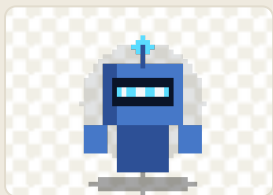
inimigo-sentinel.png
