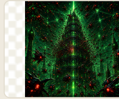
fase-ddos-enxame.png
