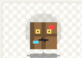
inimigo-pacote.png
