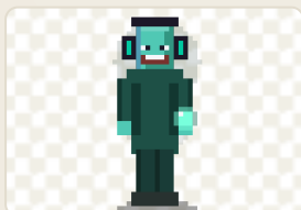
heroi-xeno.png
