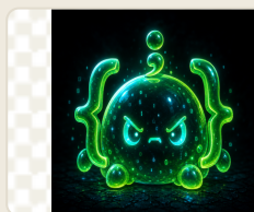
fase-primeiros-passos.png
