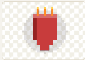
item-egide.png
