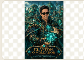
mestre-clayton.png
