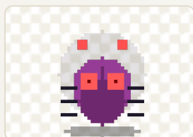
inimigo-bug.png
