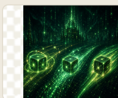
fase-tcp-udp-http.png
