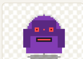
inimigo-godclass.png
