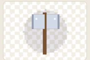
item-machado.png
