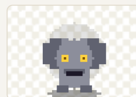
inimigo-gargula.png
