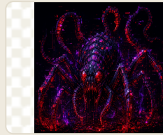
fase-bug-primordial.png
