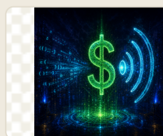
fase-variaveis-eco.png
