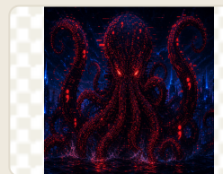
fase-parse-error-kraken.png
