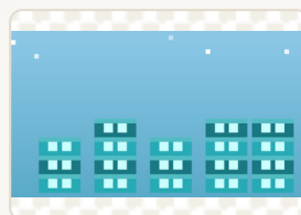
fundo-cidadela.png
