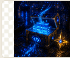
fase-bau-select.png
