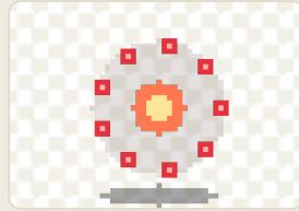
inimigo-ddos.png
