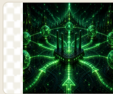
fase-ip-dns-rotas.png
