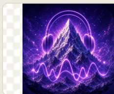
fase-montanha-chegada.png
