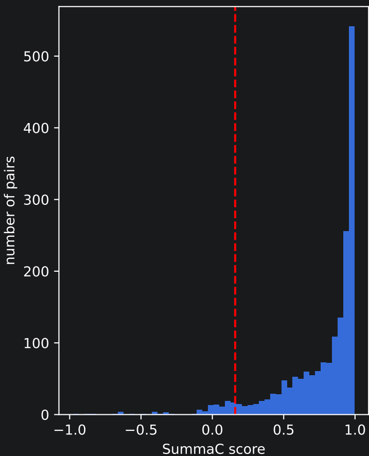
v2 Forward score
