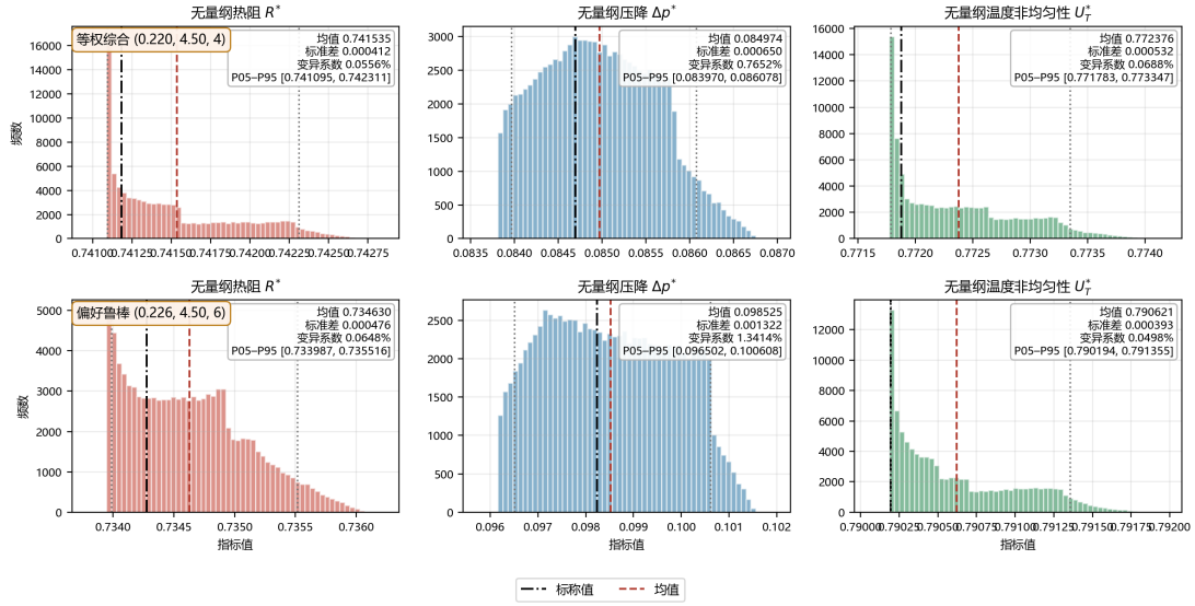
图 10 有界制造误差下两方案三项性能指标的蒙特卡洛分布 ( \beta \pm 0.01 、 \lambda \pm 0.05 , 100000 次抽样)
