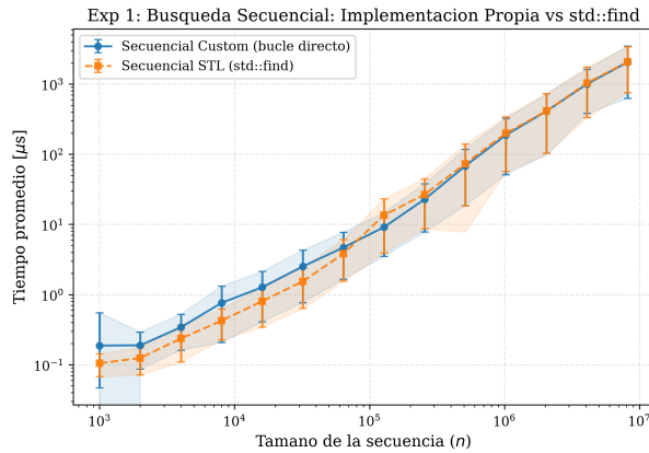
(a) Secuencial Custom vs std::find .
