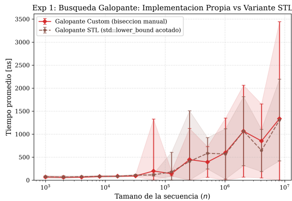
(c) Galopante Custom vs Variante STL.
