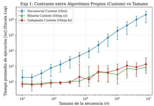
(d) Contraste Global entre Algoritmos Propios.
