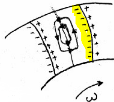
Figura 8.6: Perdita per effetto slip
