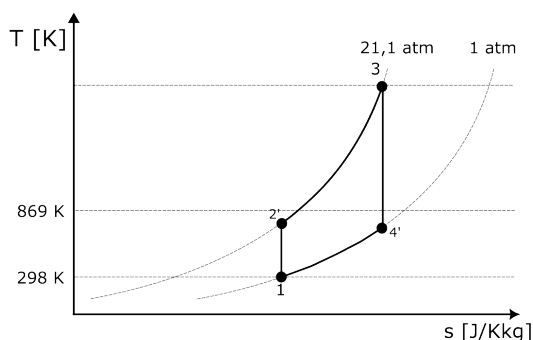
(a) Ciclo limite
