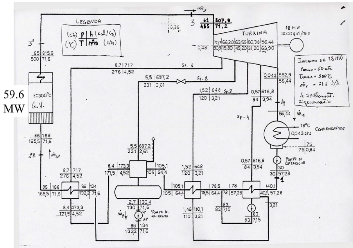
Figura 2.6: Schema di un impianto a vapore che segue ciclo a vapore surriscaldato con più di uno spillamento
