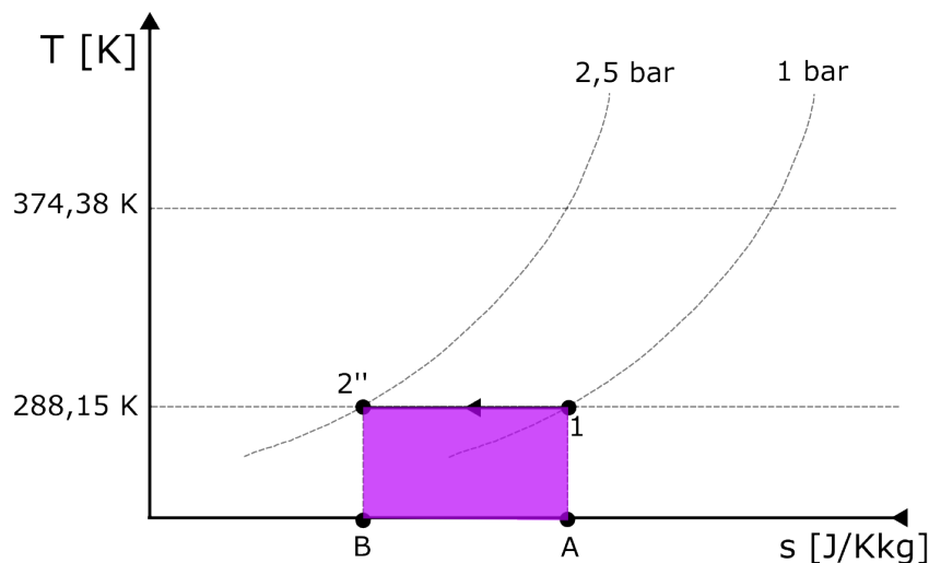
Figura 1.5: L' area B2''1A (in viola) rappresenta sia il lavoro che devo fornire sia il calore che devo sottrarre
