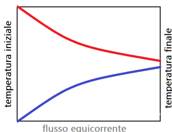
Figura 2.8: Profilo equivalente di uno scambiatore a miscela
