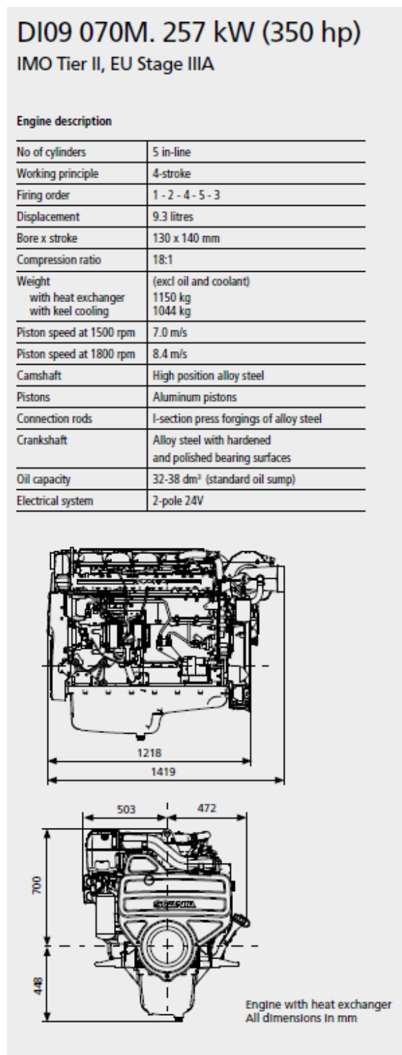
Figura 6.4: Caratteristiche principali del motore DI09 070M. 257 kW (Scania) per la propulsione navale.
