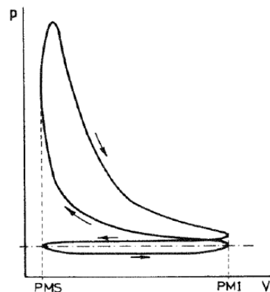
Figura 6.2: Diagramma indicato di un motore a quattro tempi in coordinate pV
