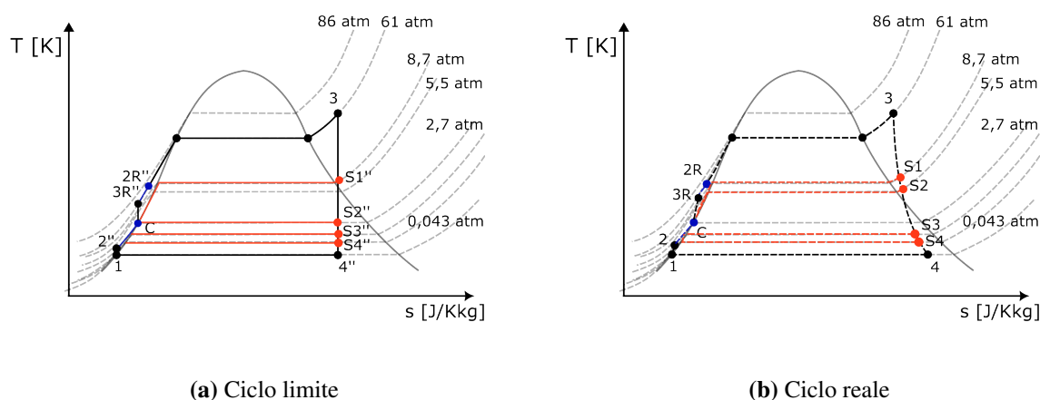
Figura 2.7: Ciclo limite e reale, con rappresentazione dello spillamento
