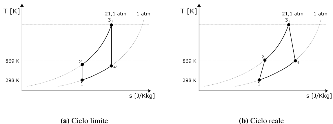
Figura 3.8: Cicli Joule limite e reale di una turbina gas
