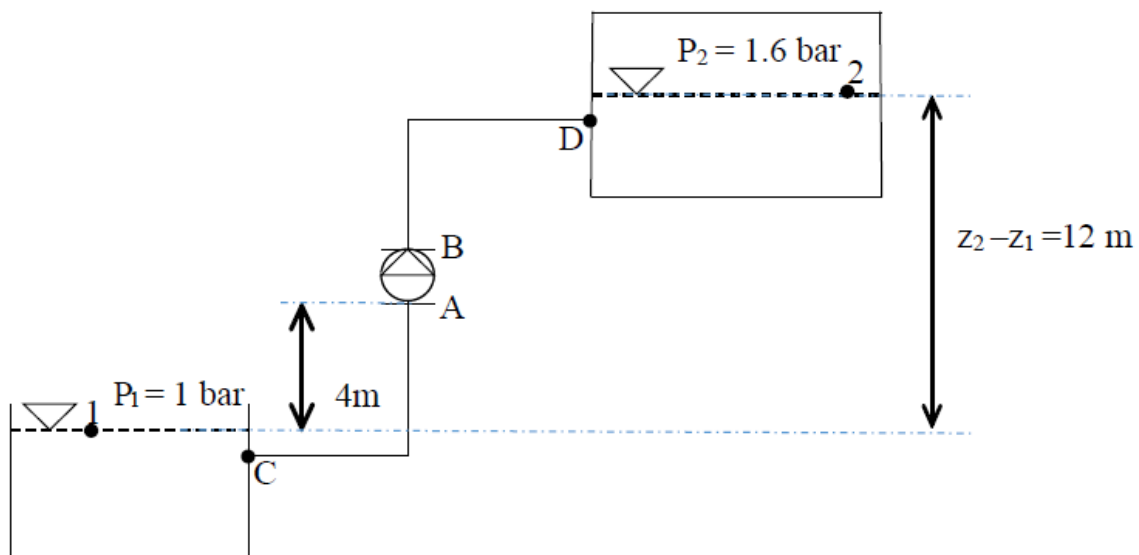
Figura 8.1: Circuito idraulico in cui è stata inserita una pompa centrifuga
