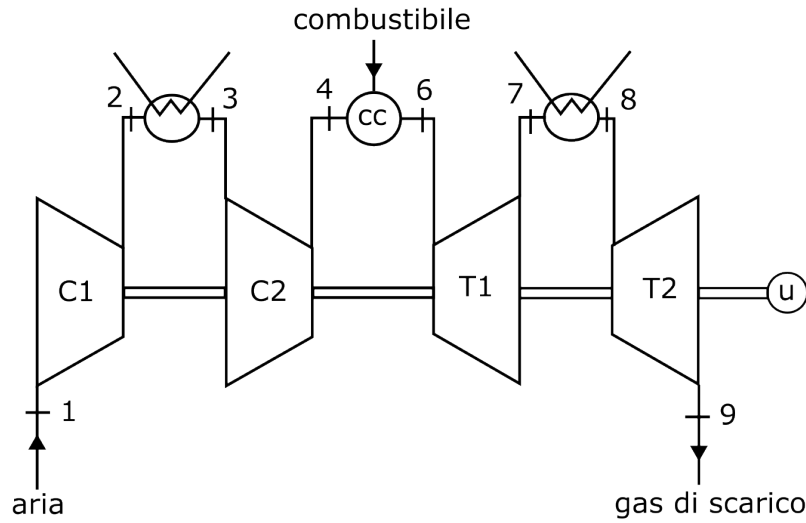
Figura 3.5: Schema dell'impianto
