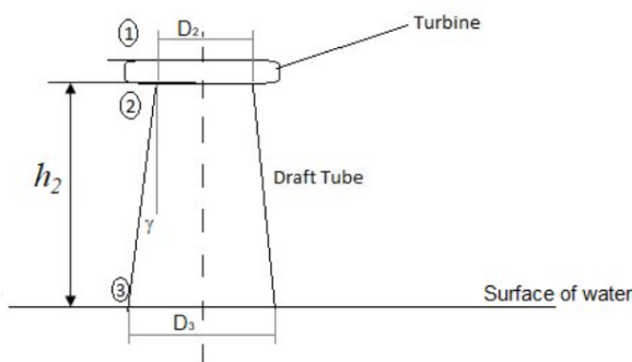
Figura 7.4: Schema di un diffusore
