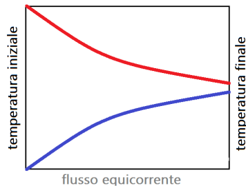
Figura 2.8: Profilo equivalente di uno scambiatore a miscela
