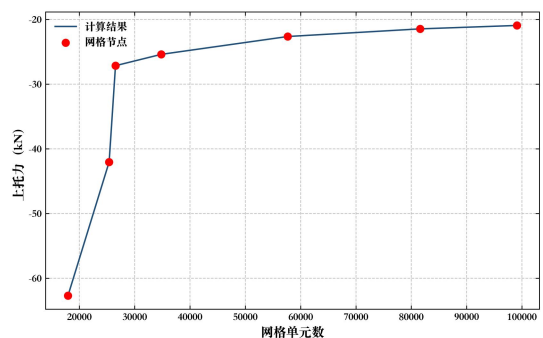
图3 网格无关性验证曲线图
