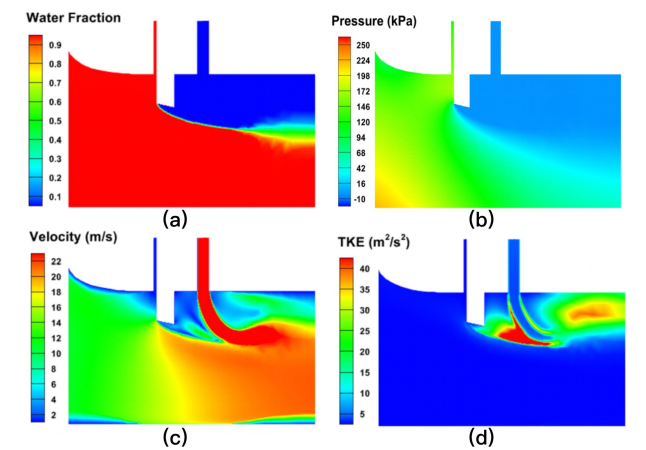
图 5 开度 0.75 工况局部流场特性云图: (a) 气液相分布; (b) 压力分布; (c) 速度分布; (d) 湍动能分布
