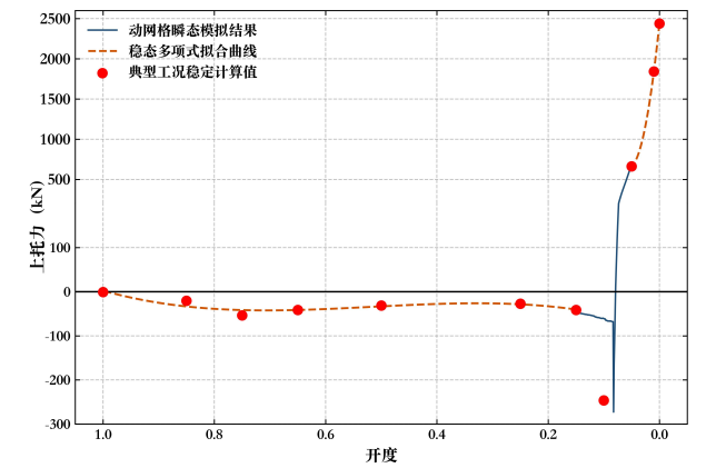
图 4 上托力与开度变化曲线及分段拟合结果
