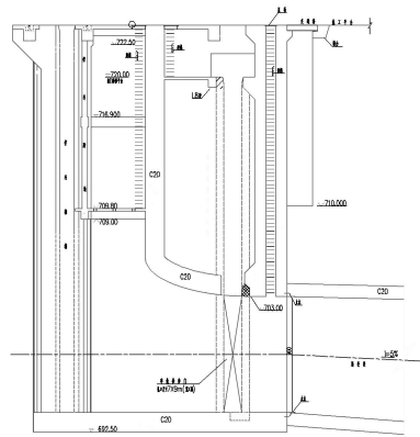
图1 水工设计总图 (单位: mm)
