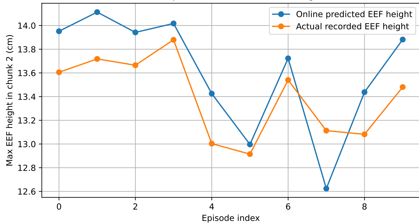
Online predicted vs actual EEF height
