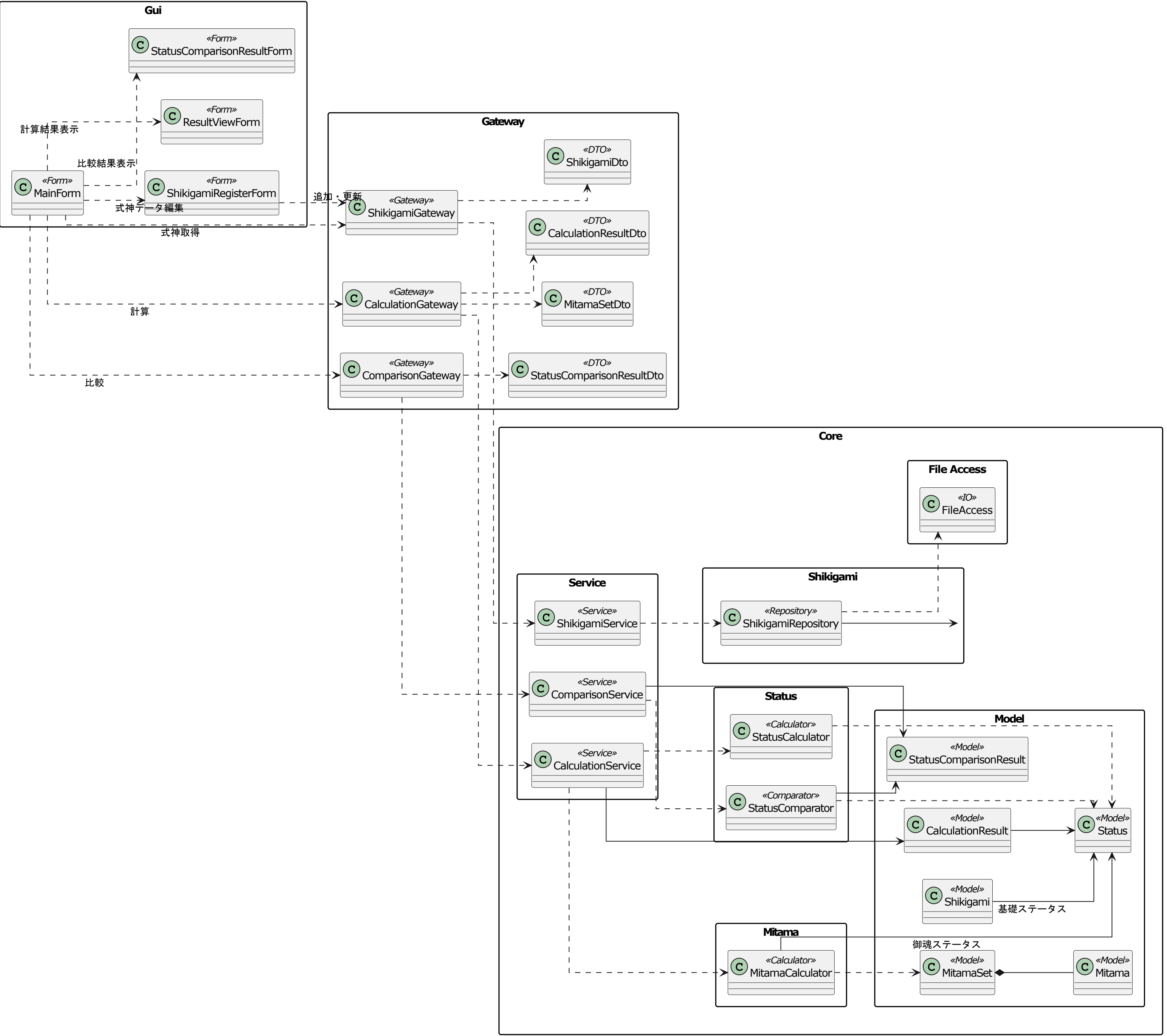
ShikigamiApp 主要クラス図
