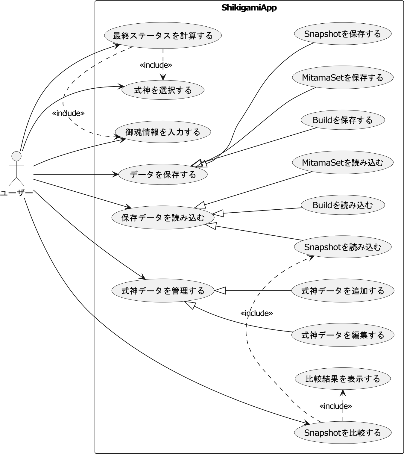
ShikigamiApp ユースケース図
