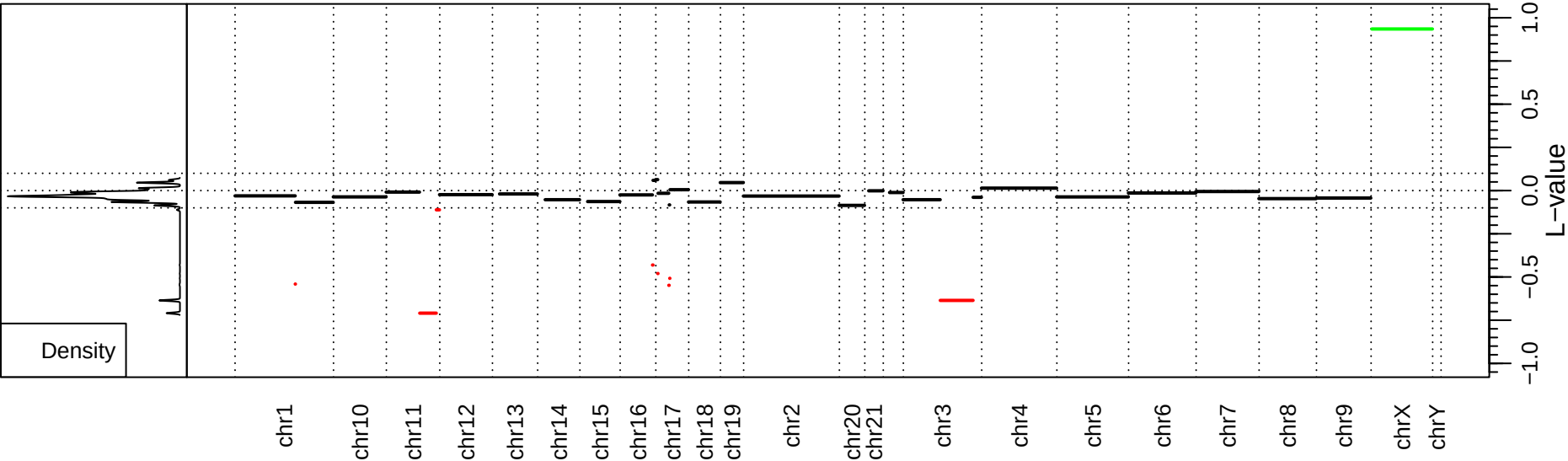
Sample:: 203219650162_R08C01
