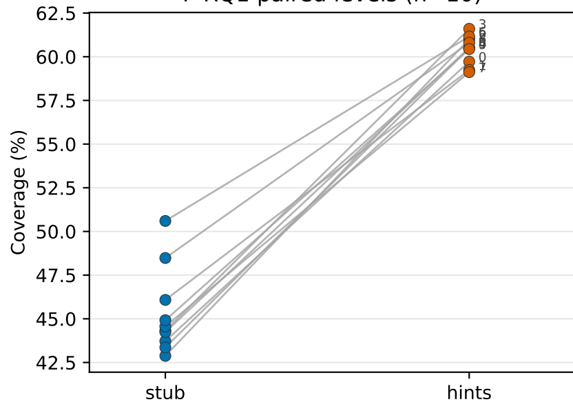
F-RQ1 paired levels (n=10)
