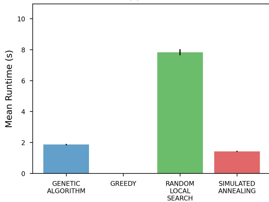
(d) Runtime
