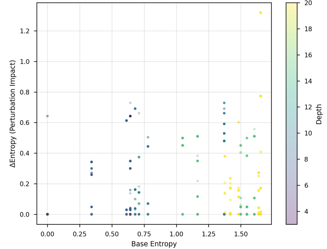
(d) Base Entropy vs Perturbation Impact Pearson r=0.2521
