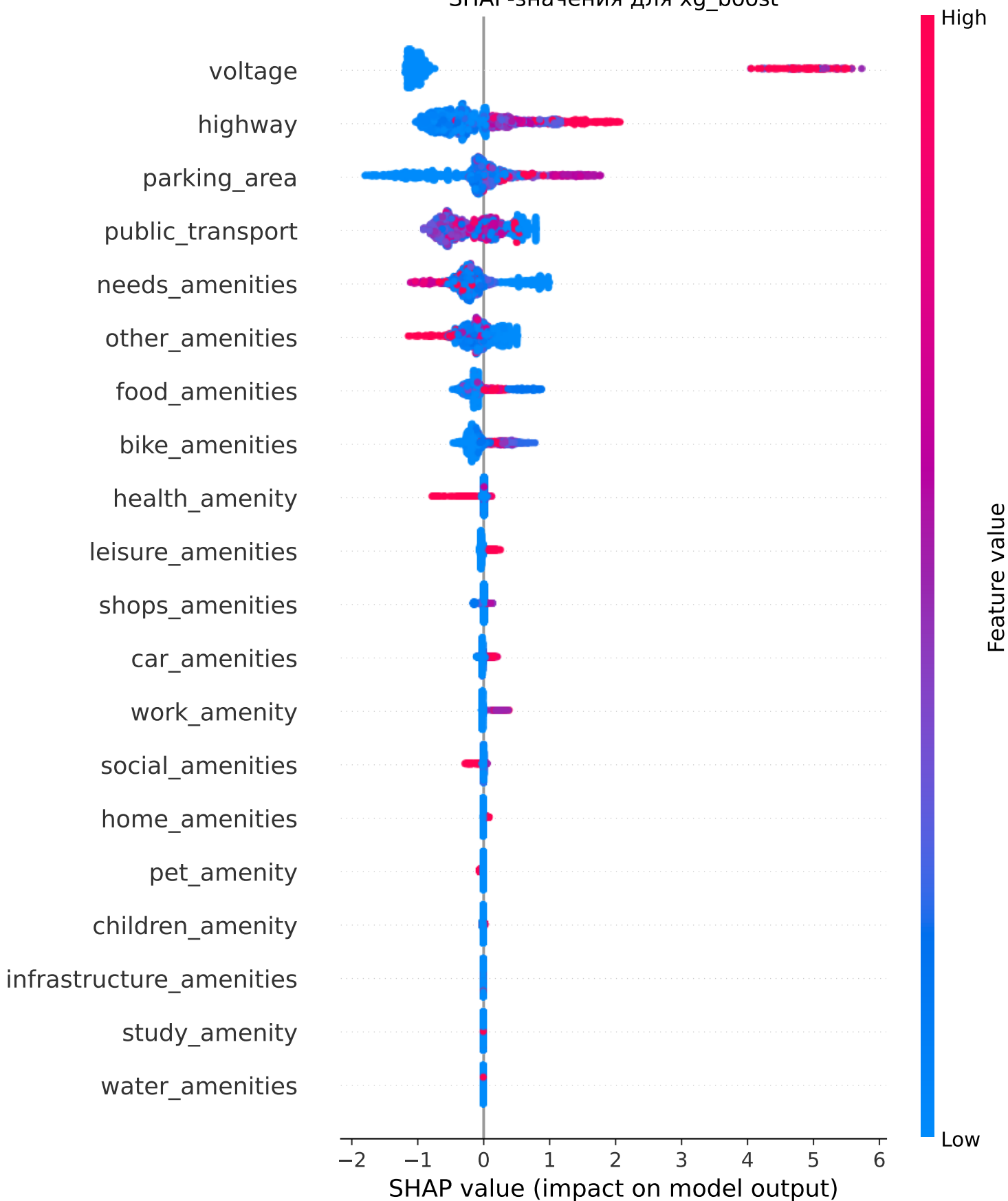
SHAP-значения для xg_boost
