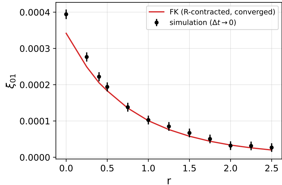
\xi_{01}(r, t = 3.48)
