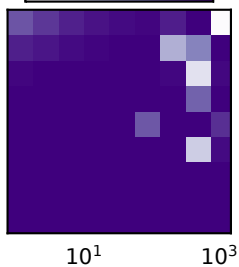
\psi_{res}
