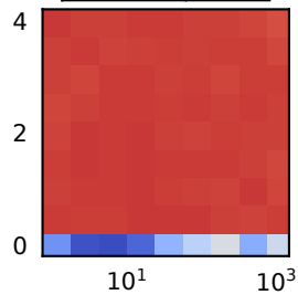
g_{0,E \rightarrow \emptyset} 0.0 0.5
