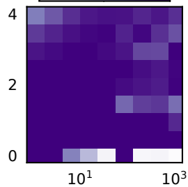
\psi_E -1 0 1
