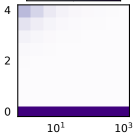
\psi_I -1 0 1
