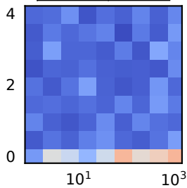
g_{0,N^* \rightarrow E} 0.0 0.5
