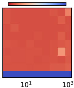
g_{0,E \rightarrow \emptyset}
