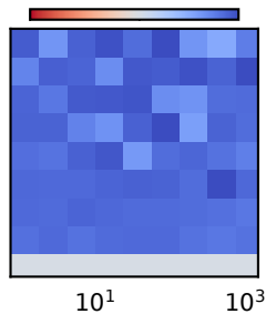
g_{0,N^* \rightarrow E}
