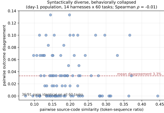
图 1: 语法多样性与行为坍缩 (Phase I, 发现研究)。首日 14 个 harness、60 道题, 91 对含 bare 和 react。每点为一对: 横轴是 token 序列代码相似度, 纵轴是正确性不同的题目比例; \rho = -0.01 , 36/91 对在全 60 题上相同。原始点见代码材料中的 fig1_phenomenon_data.json 。
