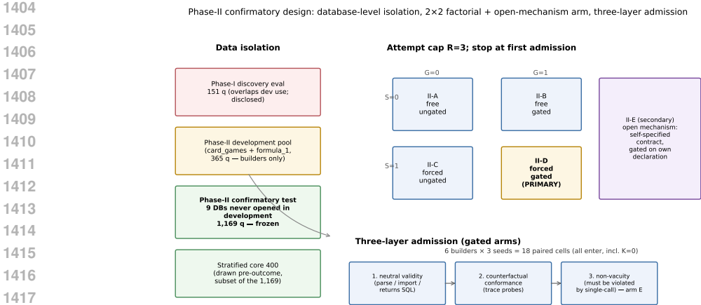
图 3: Phase-II 验证性设计（冻结协议）。左：数据库级污染隔离。中：2x2 析因与共同尝试上限，加开放机制臂 II-E。右：三层准入流程。
