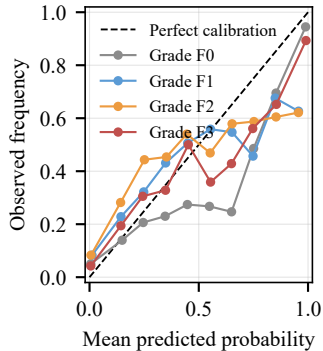
(d) Reliability, SynAP-Fib (E)
